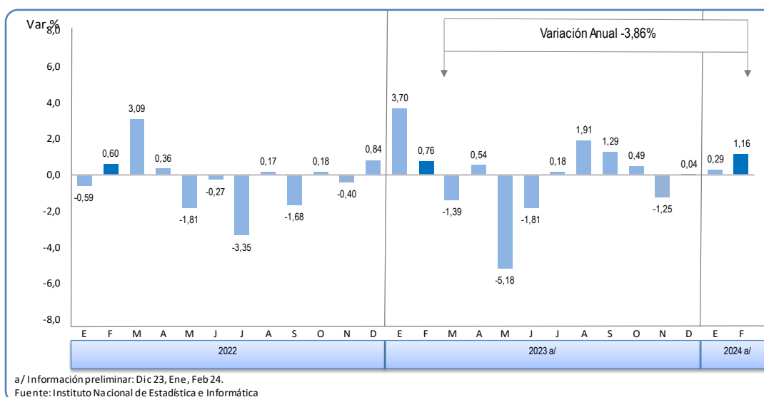
VARIACIÓN PORCENTUAL MENSUAL DEL ÍNDICE DE PRECIOS AL PRODUCTOR ENERO 2022 - FEBRERO 2024 (Base 2015 = 100)
