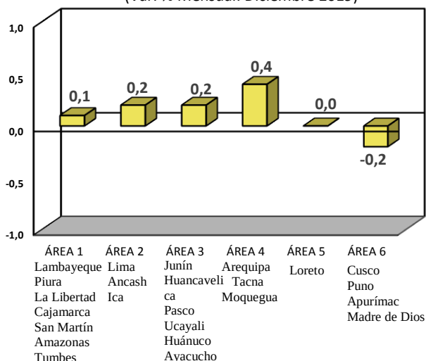
AGREGADO FINO (Var. % Mensual: Diciembre 2019)
