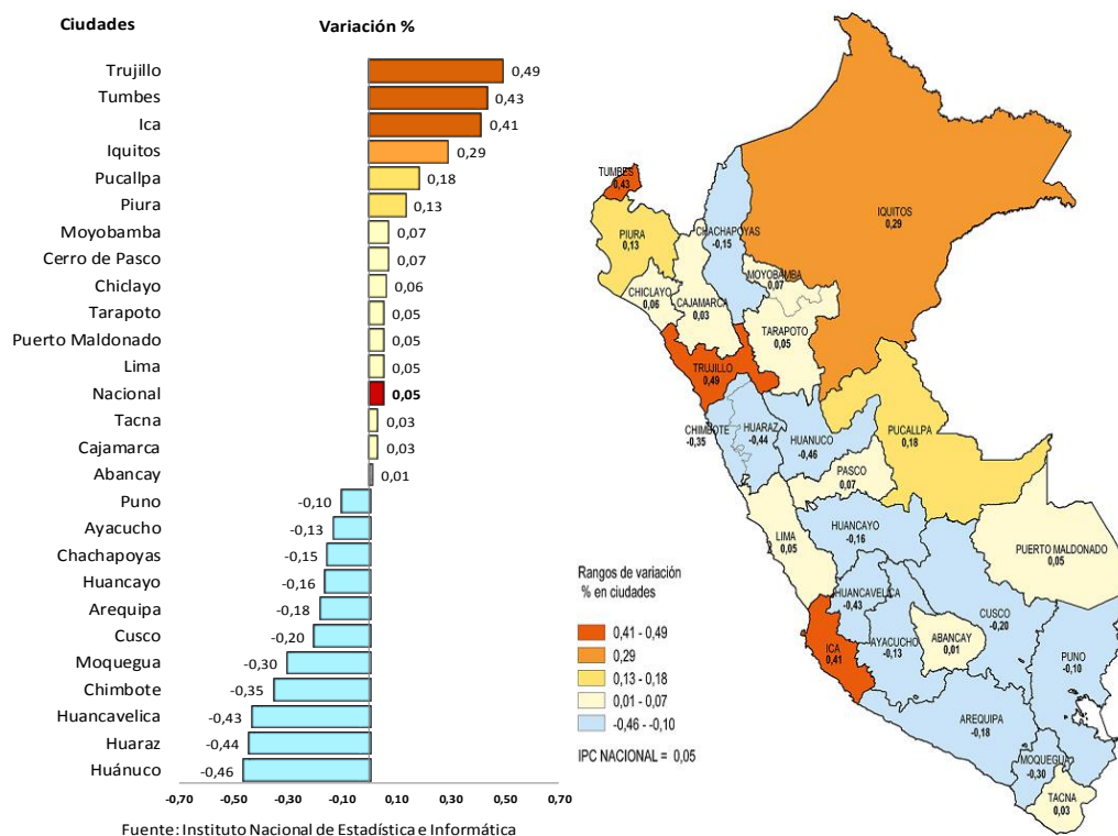
Variación Porcentual del Índice de Precios al Consumidor Nacional y de Principales Ciudades Enero 2020
