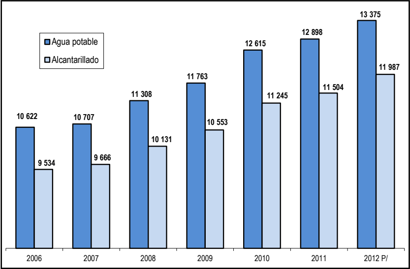
RED DE AGUA POTABLE Y ALCANTARILLADO: 2006- 2012 (Kilómetros)
