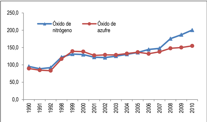
Emisiones de Óxido de nitrógeno y Óxido de azufre, 1990-2010
