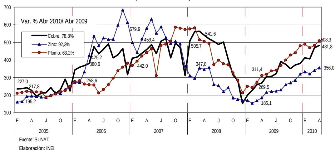
Índice Mensual de Precios de Exportación de Cobre, Zinc y Plomo: 2005-2010 (Base Año 2002=100)
