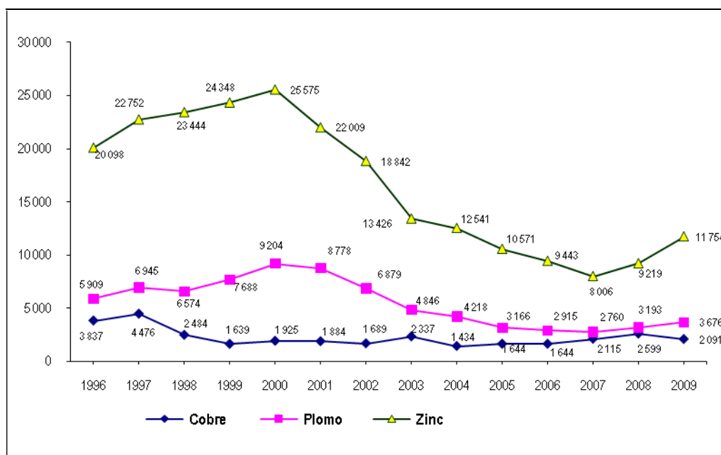
Gráfico 13.2 LA LIBERTAD: VOLUMEN DE LA PRODUCCIÓN MINERO METÁLICA, 1996 - 2009 (Tonelada métrica de contenido fino)
