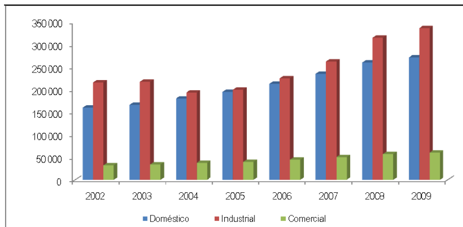
Gráfico 15.1 LA LIBERTAD: CONSUMO DE ENERGÍA ELÉCTRICA DE SERVICIO PÚBLICO, 2002 - 2009 (Megawatt hora)
