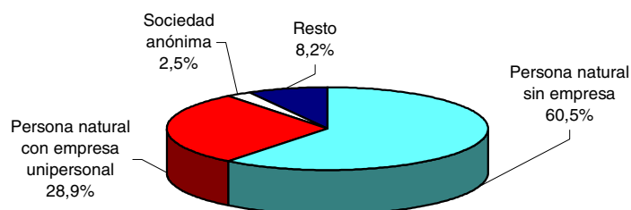
TIPO DE CONTRIBUYENTE: OCTUBRE 2001
