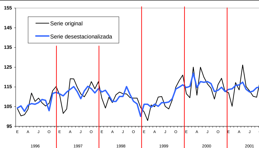
INDICE MENSUAL DEL PBI DEL SECTOR MANUFACTURA: 1996-2001 (Año base 1994=100)
