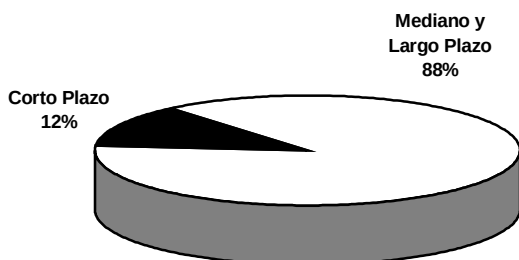
DEUDA EXTERNA TOTAL (A SETIEMBRE 2001)
