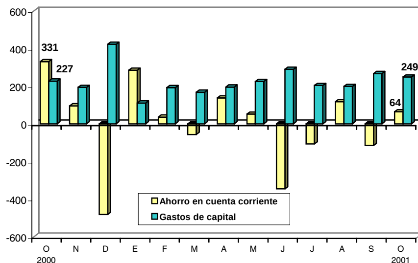
AHORRO EN CUENTA CORRIENTE Y GASTOS DE CAPITAL: 2000-2001 (Millones de nuevos soles de 1994)
