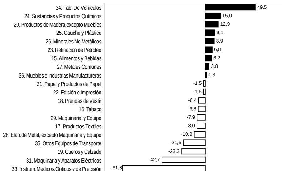
VARIACION PORCENTUAL MENSUAL DE LAS DIVISIONES INDUSTRIALES DEL SECTOR MANUFACTURERO: OCTUBRE 2001
