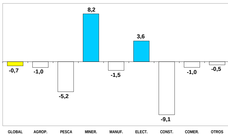
PRODUCTO BRUTO INTERNO GLOBAL Y SECTORIAL, OCTUBRE 2001 (Variación porcentual acumulada)
