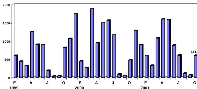
DESEMBARQUE DE LA PESCA MARITIMA: 1999-2001 (Miles de toneladas métricas brutas)
