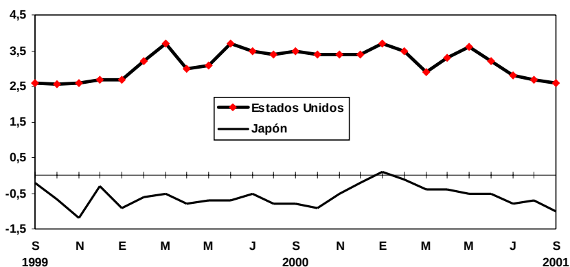
INDICE DE PRECIOS AL CONSUMIDOR DE ESTADOS UNIDOS Y JAPON: 1999-2001 (VARIACION PORCENTUAL RESPECTO A SIMILAR MES DEL AÑO ANTERIOR)
