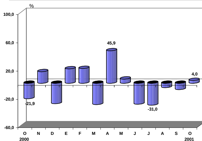
PRODUCCION DEL SECTOR PESCA: 2000-2001 (Variación porcentual referida a similar mes del año anterior)
