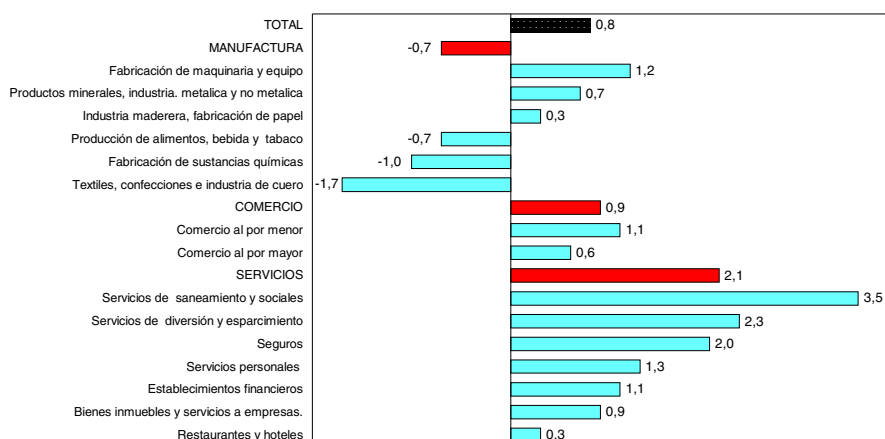
VARIACION PORCENTUAL DEL EMPLEO EN LIMA METROPOLITANA SEGUN SUBRAMA DE ACTIVIDAD ECONOMICA: SETIEMBRE / AGOSTO 2001 (Empresas de 100 y más trabajadores)
