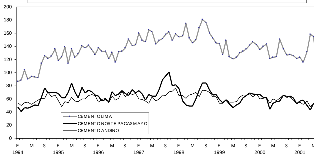
DESPACHO TOTAL DE CEMENTO: 1994 - 2001 (MILES DE TONELADAS METRICAS)
