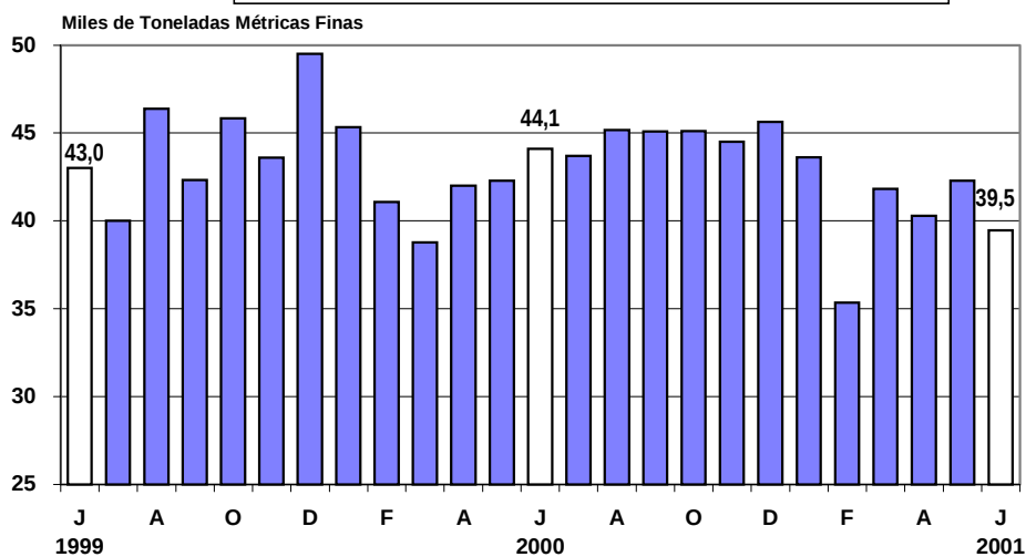
PRODUCCION DE COBRE DE LA GRAN MINERIA, 1999-2001
