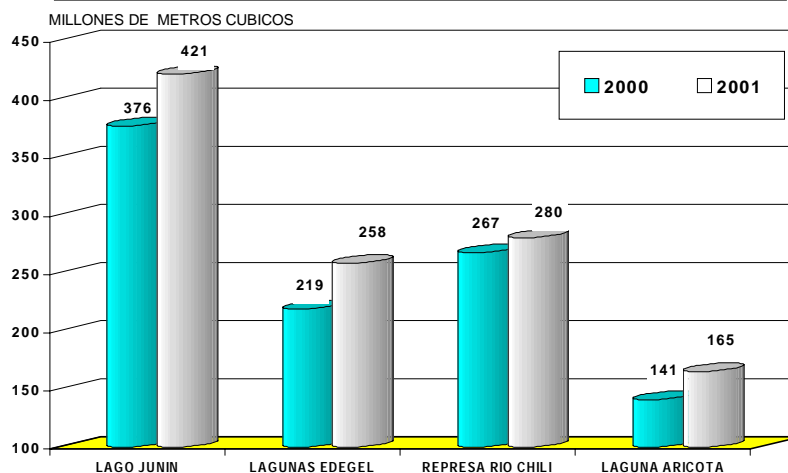
DISPONIBILIDAD DE AGUA PARA GENERACION ELECTRICA, ENERO 2000-01
