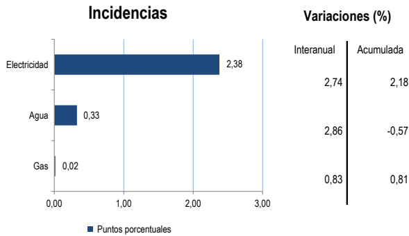
Índice de la Producción de Electricidad Gas y Agua, según actividad Año base 2007 Incidencias, variaciones interanuales y acumuladas Setiembre 2025
