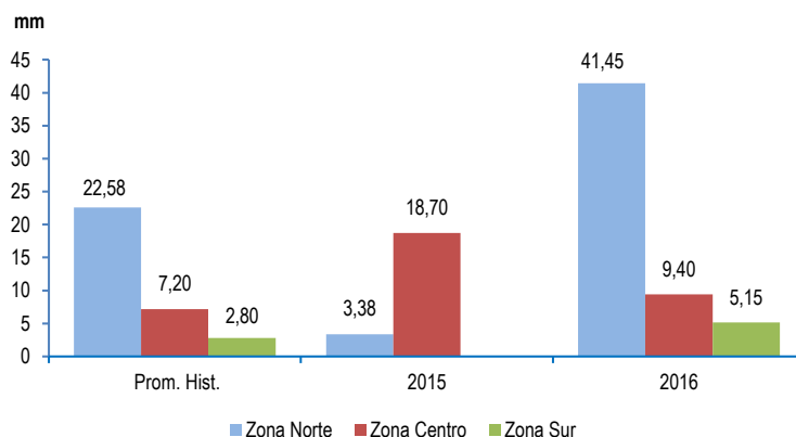
Gráfico N° 25 PERÚ: PROMEDIO DE LAS PRECIPITACIONES DE LA VERTIENTE DEL PACÍFICO, JUNIO 2015-2016
