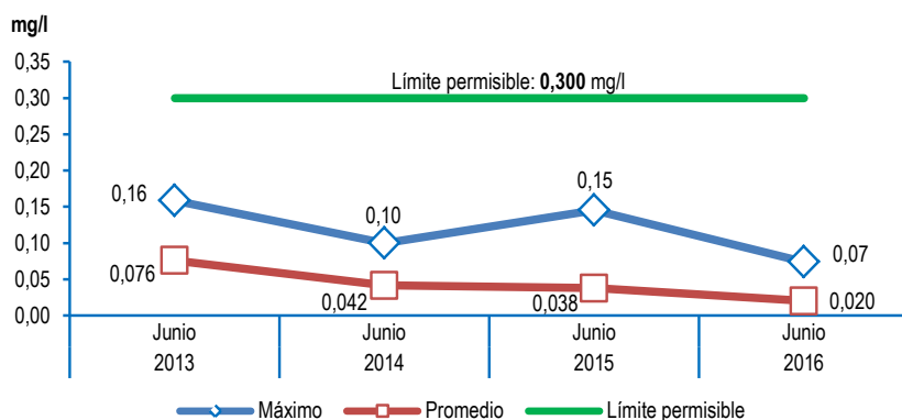
Gráfico N° 10 LIMA METROPOLITANA: CONCENTRACIÓN DE HIERRO (Fe) EN LAS PLANTAS DE TRATAMIENTO 1 Y 2 DE SEDAPAL, JUNIO 2013-2016
