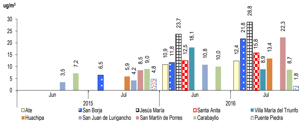
Gráfico N° 05 LIMA METROPOLITANA: VALOR DE OZONO TROPOSFÉRICO (O 3 ), POR ESTACIONES DE MEDICIÓN, 2015-2016 (µg/m 3 )
