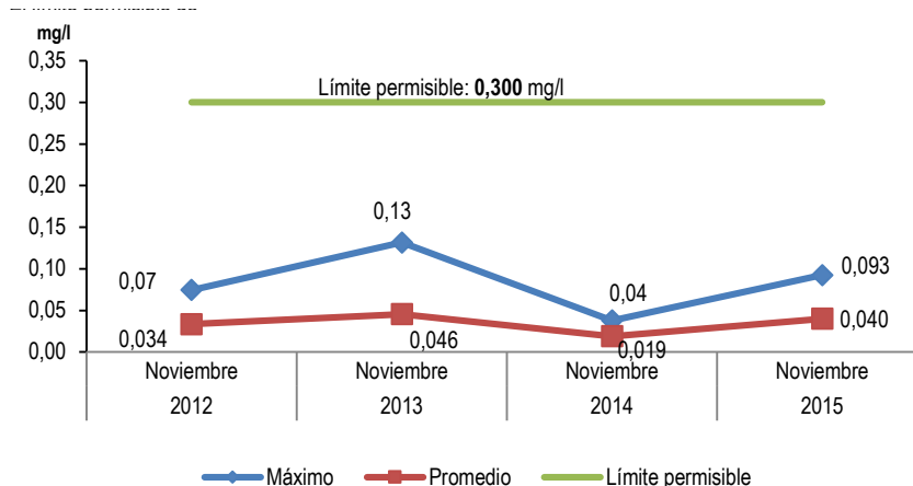
Gráfico N° 06 LIMA METROPOLITANA: CONCENTRACIÓN DE HIERRO (Fe) EN LAS PLANTAS DE TRATAMIENTO 1 Y 2 DE SEDAPAL, NOVIEMBRE 2012-2015
