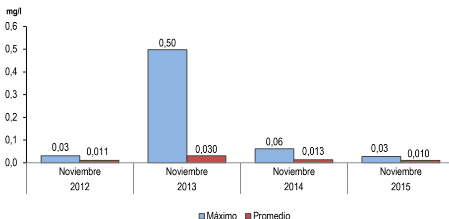
Gráfico N° 07 LIMA METROPOLITANA: CONCENTRACIÓN DE PLOMO (Pb) EN EL RÍO RÍMAC, NOVIEMBRE 2012-2015
