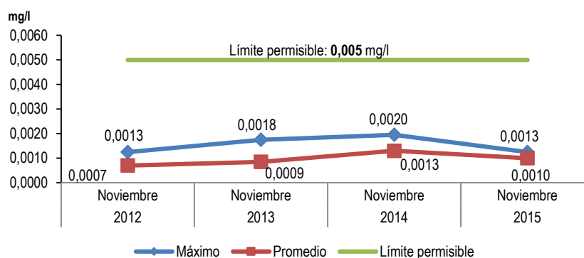
Gráfico N° 10 LIMA METROPOLITANA: CONCENTRACIÓN DE CADMIO (Cd) EN LAS PLANTAS DE TRATAMIENTO 1 Y 2 DE SEDAPAL, NOVIEMBRE 2012-2015
