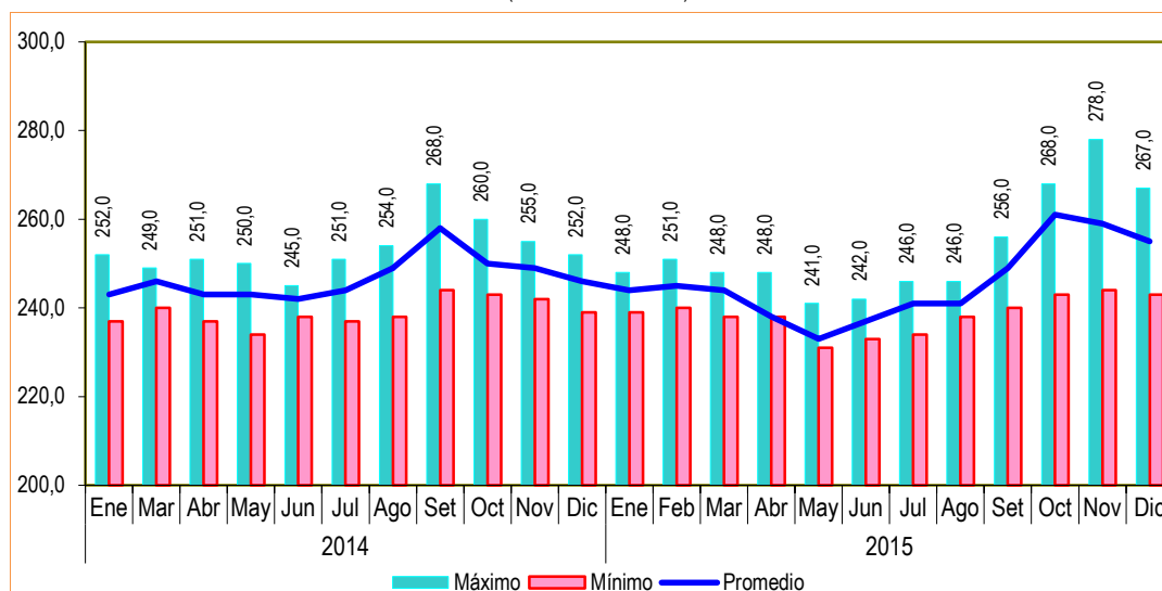
Gráfico N° 04 PERÚ: VIGILANCIA DE LA ATMÓSFERA GLOBAL, EN LA ESTACIÓN MARCAPOMACOCOA, 2014-2015 (Unidad Dobson -UD)
