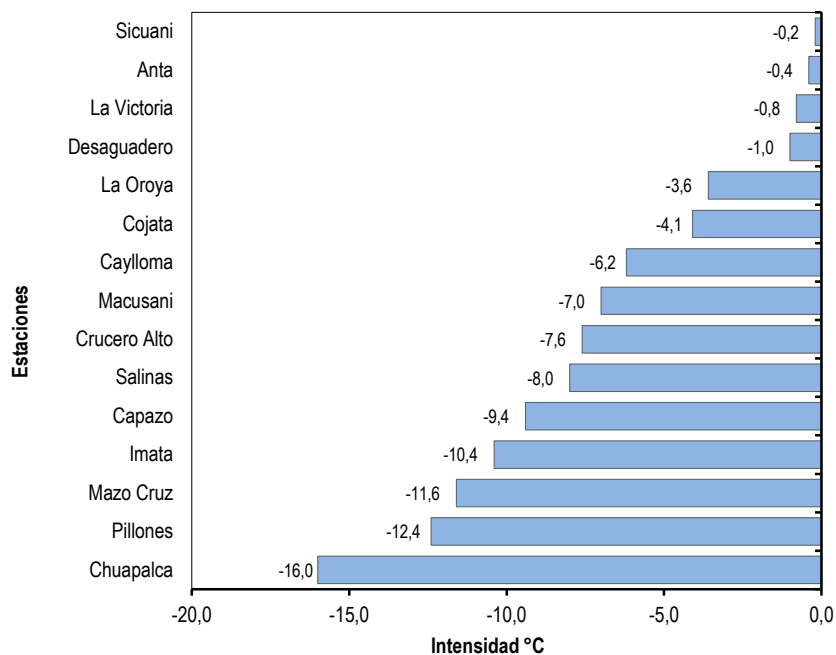
Gráfico N° 27 PERÚ: INTENSIDAD DE LAS HELADAS METEOROLÓGICAS, NOVIEMBRE 2015 (Temperatura bajo cero grados)
