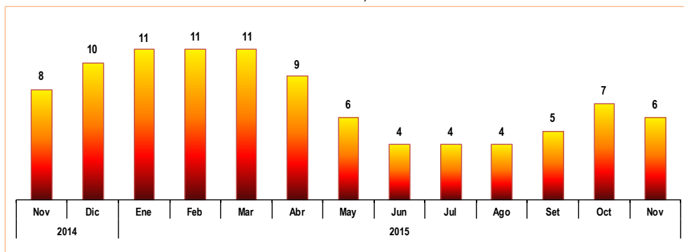
LIMA METROPOLITANA: ÍNDICE UV-B PROMEDIO MENSUAL, 2014-2015
