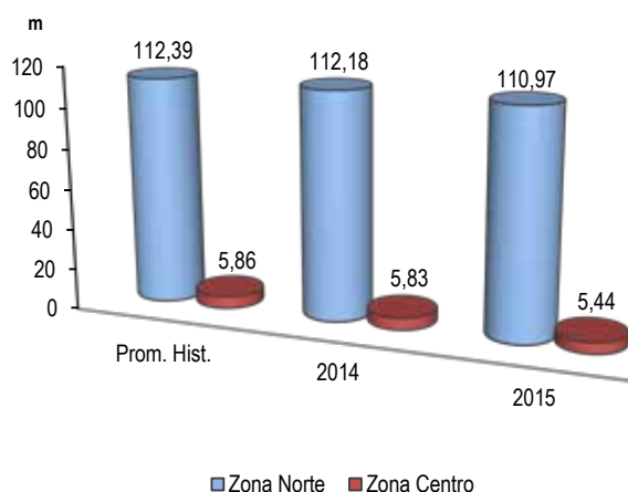
Gráfico N° 22 PERÚ: CAUDAL PROMEDIO DE LOS RÍOS DE LA VERTIENTE DEL ATLÁNTICO, NOVIEMBRE 2014-2015
