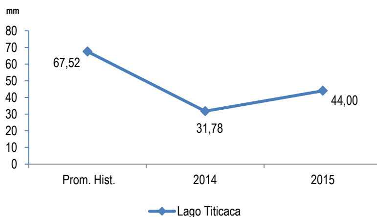
Gráfico N° 26 PERÚ: PROMEDIO DE LAS PRECIPITACIONES DE LA VERTIENTE DEL LAGO TITICACA, NOVIEMBRE 2014-2015
