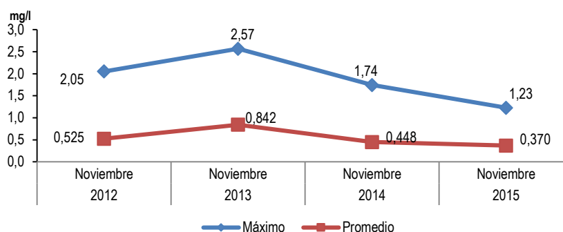
Gráfico N° 11 LIMA METROPOLITANA: CONCENTRACIÓN DE ALUMINIO (Al) EN EL RÍO RÍMAC, NOVIEMBRE 2012-2015
