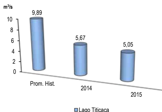
Gráfico N° 23 PERÚ: CAUDAL PROMEDIO DE LOS RÍOS DE LA VERTIENTE DEL LAGO TITICACA, NOVIEMBRE 2014-2015
