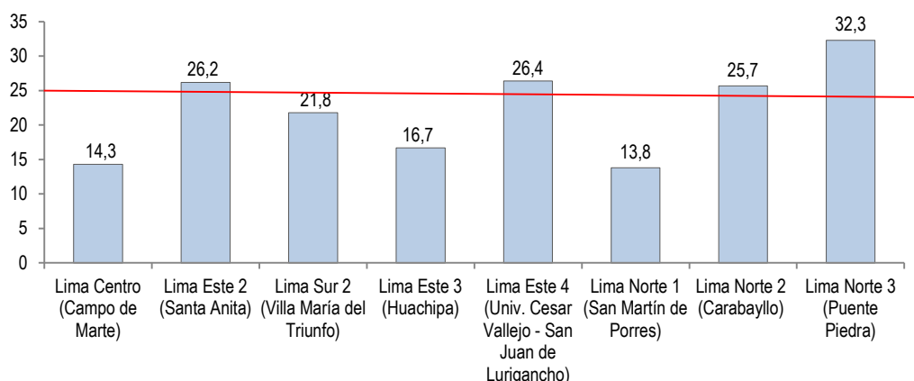
Gráfico N° 02 LIMA METROPOLITANA: CONCENTRACIÓN DE PARTÍCULAS INFERIORES A 2,5 MICRAS (PM 2,5 ), DICIEMBRE 2015
