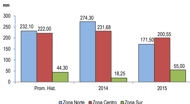
Gráfico N° 25 PERÚ: PROMEDIO DE LAS PRECIPITACIONES DE LA VERTIENTE DEL ATLÁNTICO, NOVIEMBRE 2014-2015
