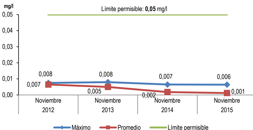
Gráfico N° 08 LIMA METROPOLITANA: CONCENTRACIÓN DE PLOMO (Pb) EN LAS PLANTAS DE TRATAMIENTO 1 Y 2 DE SEDAPAL, NOVIEMBRE 2012-2015
