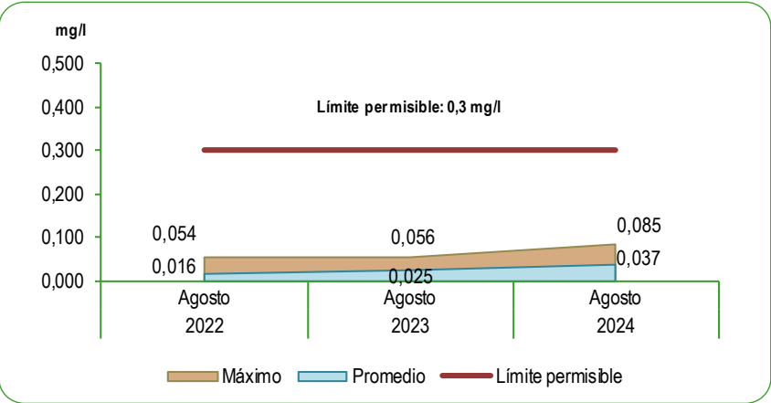
GRÁFICO N°34 LIMA METROPOLITANA: CONCENTRACIÓN DE HIERRO (Fe) EN LAS PLANTAS DE TRATAMIENTO 1 Y 2 DE SEDAPAL Agosto 2022 - 2024 Miligramos por litro (mg/l)
