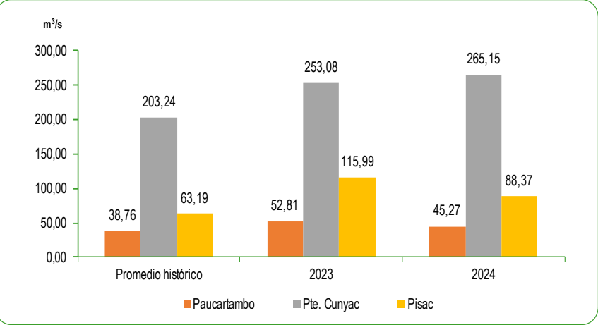
GRÁFICO N°54 PERÚ: CAUDAL PROMEDIO DE LOS RÍOS DE LA ZONA SUR DE LA VERTIENTE DEL ATLÁNTICO Diciembre2023 - 2024 Metro cúbico por segundo (m³/s)
