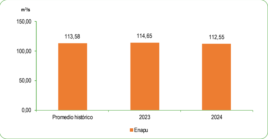
GRÁFICO N°52 PERÚ: CAUDAL PROMEDIO DE LOS RÍOS DE LA ZONA NORTE DE LA VERTIENTE DEL ATLÁNTICO Diciembre2023 – 2024 Metro cúbico por segundo (m³/s)
