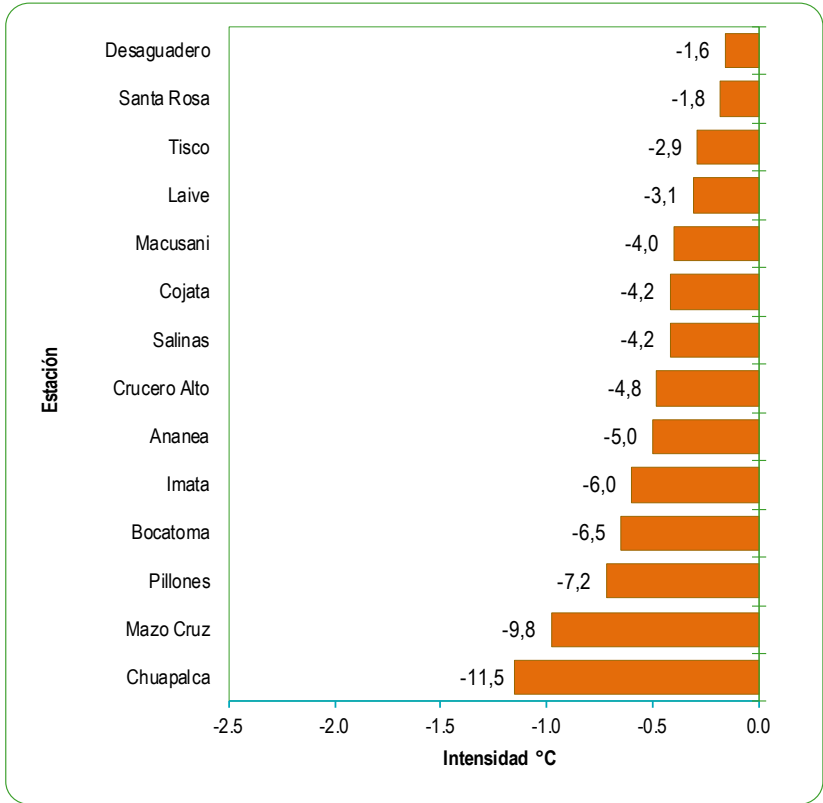
GRÁFICO N°65 PERÚ: MAYOR INTENSIDAD REGISTRADA DE LAS HELADAS METEOROLÓGICAS DICIEMBRE 2024 Temperatura bajo cero grados
