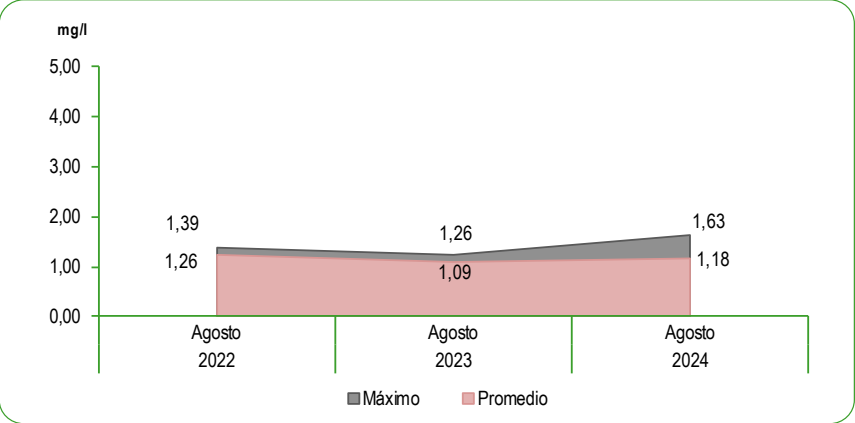
GRÁFICO N°42 LIMA METROPOLITANA: CONCENTRACIÓN DE MATERIA ORGÁNICA EXPRESADA COMO TOC EN LAS PLANTAS DE TRATAMIENTO 1 Y 2 DE SEDAPAL Agosto 2022 - 2024 Miligramos por litro (mg/l)
