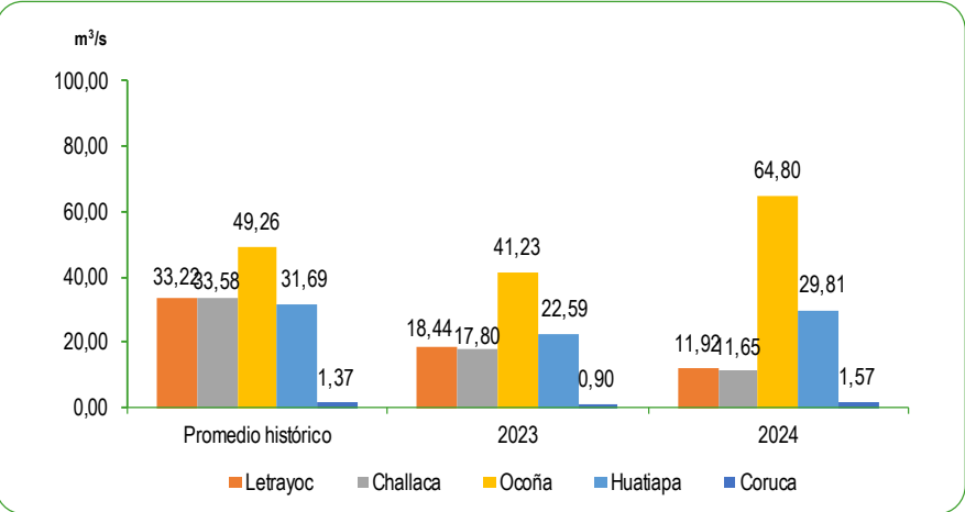
GRÁFICO N°51 PERÚ: CAUDAL PROMEDIO DE LOS RÍOS DE LA ZONA SUR DE LA VERTIENTE DEL PACÍFICO Diciembre2023 – 2024 Metro cúbico por segundo (m³/s)
