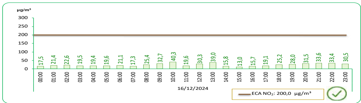
GRÁFICO N°21 LIMA METROPOLITANA: VALOR DIARIO DEL DIÓXIDO DE NITRÓGENO (NO 2 ), EN LA ESTACIÓN DE MEDICIÓN DE CAMPO DE MARTE – DICIEMBRE 2024
