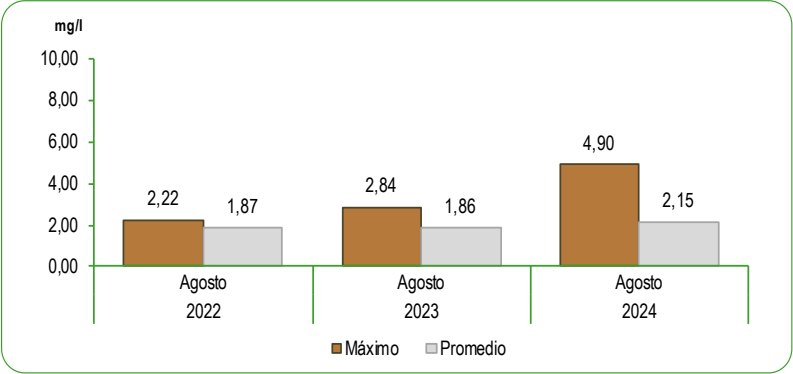
GRÁFICO N°41 LIMA METROPOLITANA: CONCENTRACIÓN DE MATERIA ORGÁNICA EXPRESADA COMO TOC EN EL RÍO RÍMAC Agosto 2022 - 2024 Miligramos por litro (mg/l)
