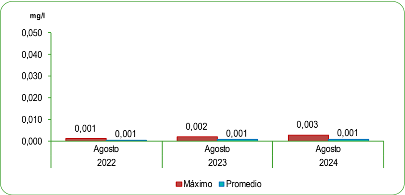
GRÁFICO N°37 LIMA METROPOLITANA: CONCENTRACIÓN DE CADMIO (Cd) EN EL RÍO RÍMAC Agosto 2022 - 2024 Miligramos por litro (mg/l)
