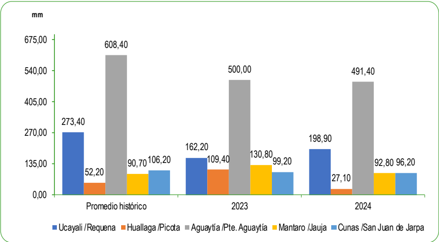
GRÁFICO N°60 PERÚ: PROMEDIO DE LAS PRECIPITACIONES EN LA ZONA CENTRO DE LA VERTIENTE DEL ATLÁNTICO Diciembre2023 - 2024 Milímetros (mm)
