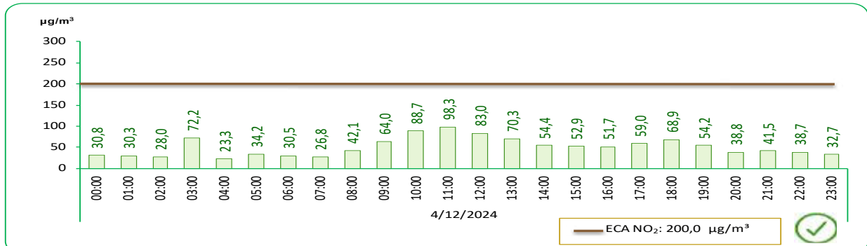
GRÁFICO N°22 LIMA METROPOLITANA: VALOR DIARIO DEL DIÓXIDO DE NITRÓGENO (NO 2 ), EN LA ESTACIÓN DE MEDICIÓN DE SAN JUAN DE LURIGANCHO – DICIEMBRE 2024
