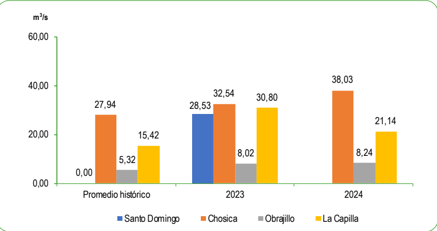
GRÁFICO N°50 PERÚ: CAUDAL PROMEDIO DE LOS RÍOS DE LA ZONA CENTRO DE LA VERTIENTE DEL PACÍFICO Diciembre2023 – 2024 Metro cúbico por segundo (m³/s)
