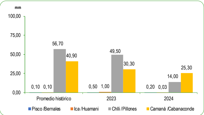
GRÁFICO N°58 PERÚ: PROMEDIO DE LAS PRECIPITACIONES EN LA ZONA SUR DE LA VERTIENTE DEL PACÍFICO Diciembre2023 - 2024 Milímetros (mm)
