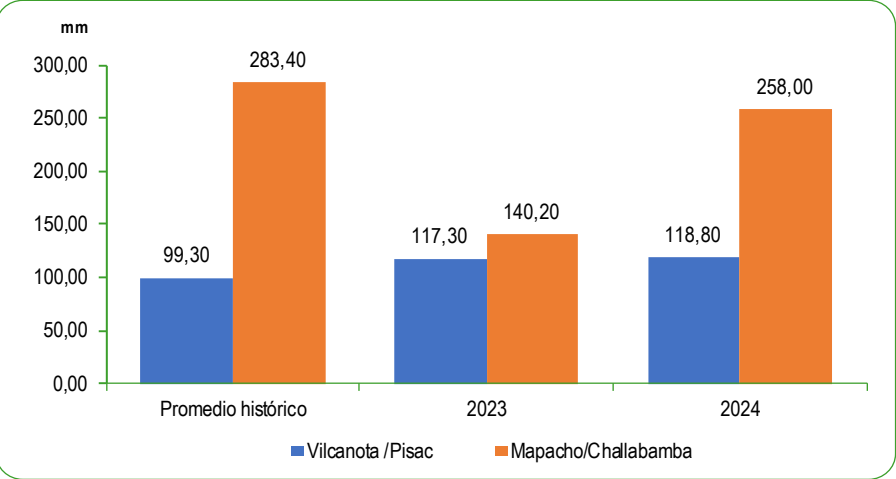
GRÁFICO N°61 PERÚ: PROMEDIO DE LAS PRECIPITACIONES EN LA ZONA SUR DE LA VERTIENTE DEL ATLÁNTICO Diciembre2023 - 2024 Milímetros (mm)
