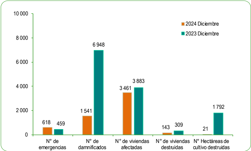
GRÁFICO N°63 PERÚ: NÚMERO DE EMERGENCIAS Y DAÑOS PRODUCIDOS A NIVEL NACIONAL Diciembre2024/ Diciembre2023 Número (N°)
