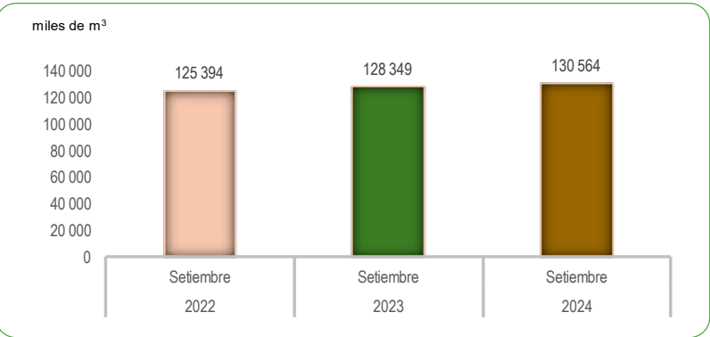
GRÁFICO N°46 PERÚ: PRODUCCIÓN NACIONAL DE AGUA POTABLE Setiembre 2022 - 2024 Miles de metros cúbicos (Miles de m³)
