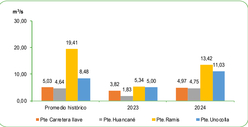
GRÁFICO N°55 PERÚ: CAUDAL PROMEDIO DE LOS RÍOS DE LA VERTIENTE DEL LAGO TITICACA Diciembre2023 – 2024 Metro cúbico por segundo (m³/s)
