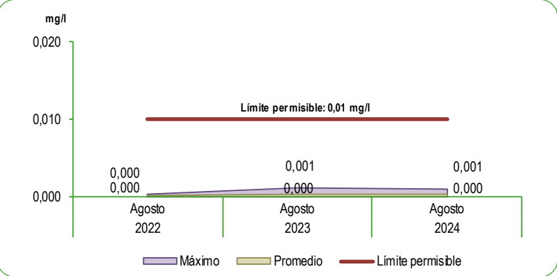
GRÁFICO N°36 LIMA METROPOLITANA: CONCENTRACIÓN DE PLOMO (Pb) EN LAS PLANTAS DE TRATAMIENTO 1 Y 2 DE SEDAPAL Agosto 2022 - 2024 Miligramos por litro (mg/l)
