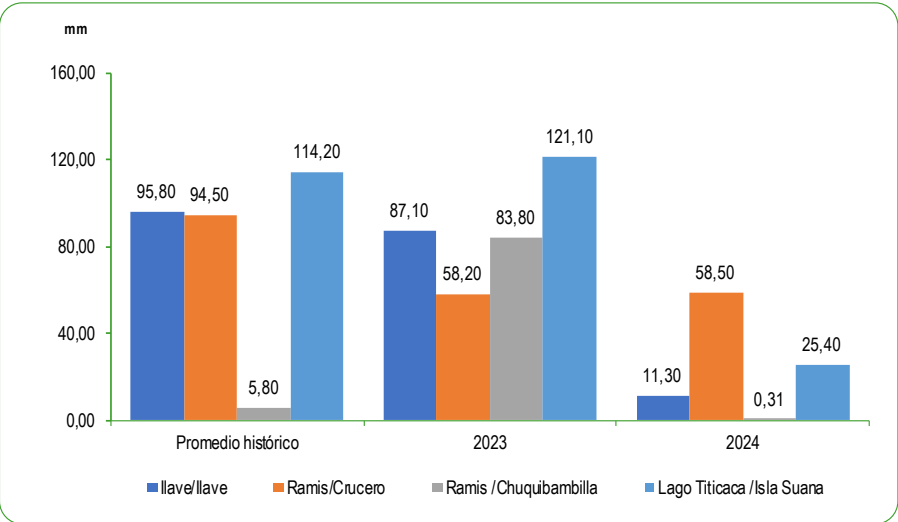
GRÁFICO N°62 PERÚ: PROMEDIO DE LAS PRECIPITACIONES EN LA VERTIENTE DEL LAGO TITICACA Diciembre2023 - 2024 Milímetros (mm)
