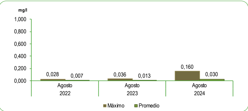
GRÁFICO N°35 LIMA METROPOLITANA: CONCENTRACIÓN DE PLOMO (Pb) EN EL RÍO RÍMAC Agosto 2022 - 2024 Miligramos por litro (mg/l)
