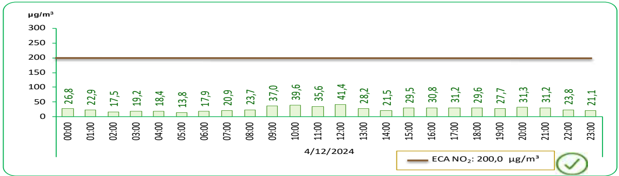
GRÁFICO N°20 LIMA METROPOLITANA: VALOR DIARIO DEL DIÓXIDO DE NITRÓGENO (NO 2 ), EN LA ESTACIÓN DE MEDICIÓN DE SAN BORJA – DICIEMBRE 2024
