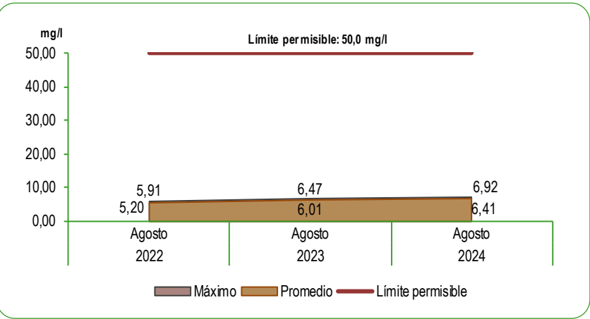
GRÁFICO N°44 LIMA METROPOLITANA: CONCENTRACIÓN DE NITRATOS (NO 3 ) EN LAS PLANTAS DE TRATAMIENTO 1 Y 2 DE SEDAPAL Agosto 2022 - 2024 Miligramos por litro (mg/l)
