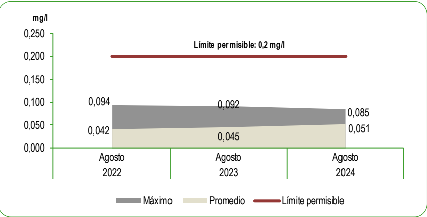
GRÁFICO N°40 LIMA METROPOLITANA: CONCENTRACIÓN DE ALUMINIO (Al) EN LAS PLANTAS DE TRATAMIENTO 1 Y 2 DE SEDAPAL Agosto 2022 - 2024 Miligramos por litro (mg/l)
