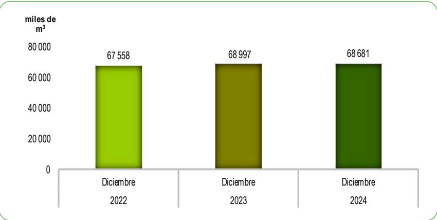
GRÁFICO N°47 LIMA METROPOLITANA: PRODUCCIÓN DE AGUA POTABLE Diciembre2022 – Diciembre2024 Miles de metros cúbicos (Miles de m³)
