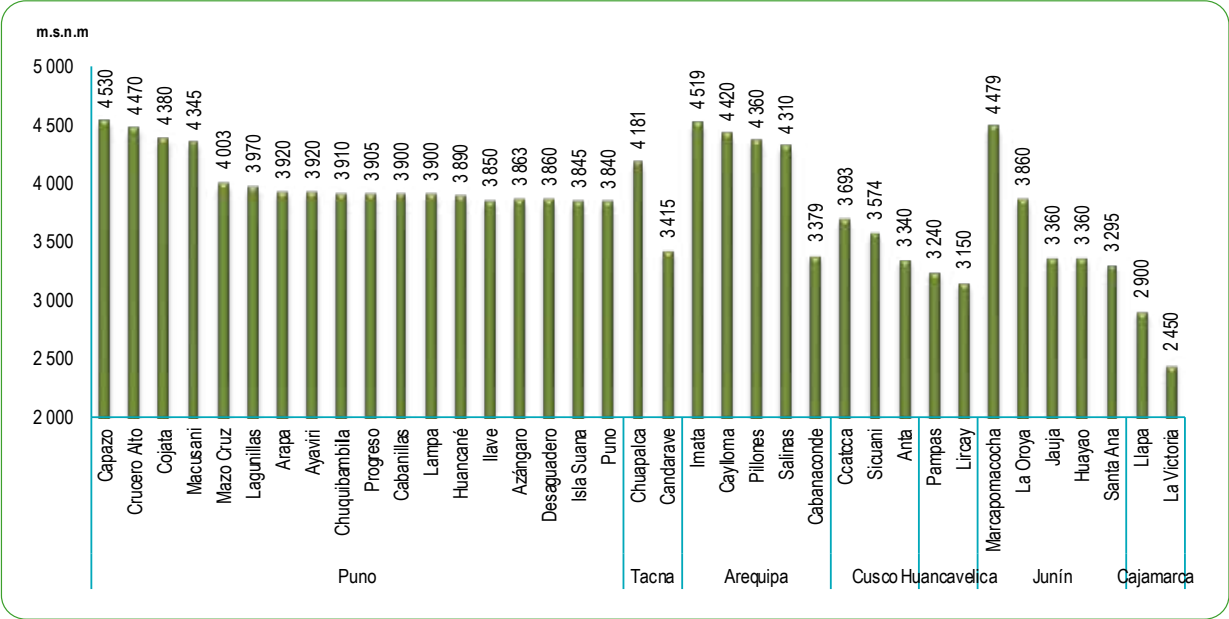
GRÁFICO N°66 PERÚ: ALTITUD DE LAS ESTACIONES METEOROLÓGICAS Metros sobre el nivel del mar
