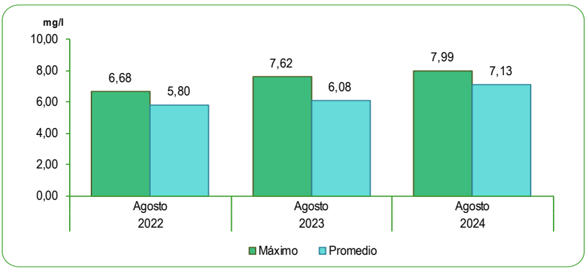
GRÁFICO N°43 LIMA METROPOLITANA: CONCENTRACIÓN DE NITRATOS (NO 3 ) EN EL RÍO RÍMAC Agosto 2022 - 2024 Miligramos por litro (mg/l)
