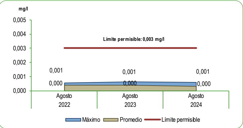
GRÁFICO N°38 LIMA METROPOLITANA: CONCENTRACIÓN DE CADMIO (Cd) EN LAS PLANTAS DE TRATAMIENTO 1 Y 2 DE SEDAPAL Agosto 2022 - 2024 Miligramos por litro (mg/l)
