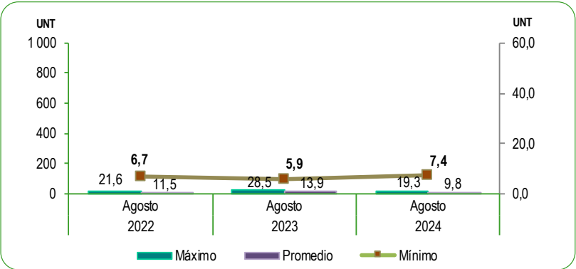
GRÁFICO N°45 LIMA METROPOLITANA: NIVELES DE TURBIEDAD EN EL RÍO RÍMAC Mes: Agosto 2022 - 2024 Unidades Nefelométricas de Turbiedad (UNT)
