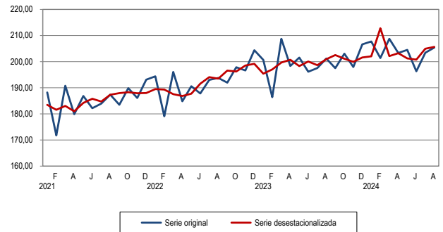
Índice de la Producción de Electricidad Gas y Agua Año base 2007 Serie original y desestacionalizada Enero 2021-Agosto 2024
