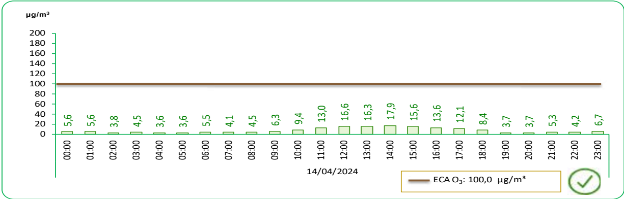
GRÁFICO N°22 LIMA METROPOLITANA: VALOR DIARIO DEL OZONO TROPOSFÉRICO (O 3 ), EN LA ESTACIÓN DE MEDICIÓN DE SAN MARTÍN DE PORRES – ABRIL 2024
