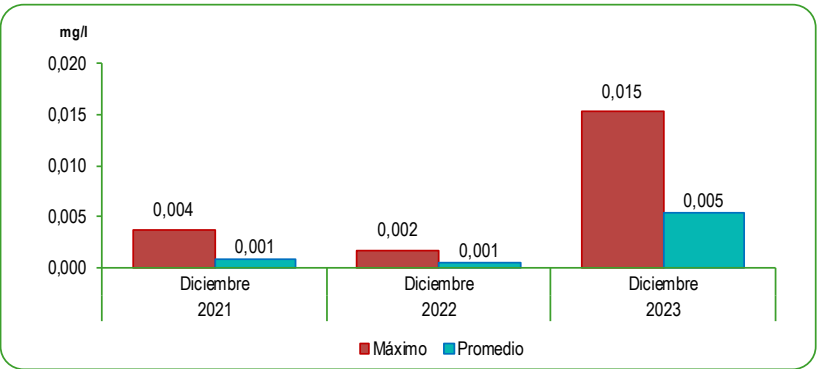
GRÁFICO N°29 LIMA METROPOLITANA: CONCENTRACIÓN DE CADMIO (Cd) EN EL RÍO RÍMAC Diciembre 2021 - 2023 Miligramos por litro (mg/l)
