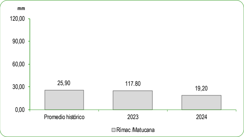
GRÁFICO N°48 PERÚ: PROMEDIO DE LAS PRECIPITACIONES EN LA ZONA CENTRO DE LA VERTIENTE DEL PACÍFICO Abril 2023 - 2024 Milímetros (mm)
