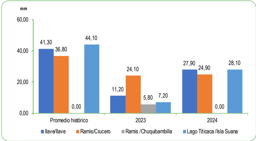
GRÁFICO N°53 PERÚ: PROMEDIO DE LAS PRECIPITACIONES EN LA VERTIENTE DEL LAGO TITICACA Abril 2023 - 2024 Milímetros (mm)
