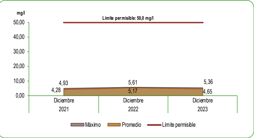
GRÁFICO N°36 LIMA METROPOLITANA: CONCENTRACIÓN DE NITRATOS (NO 3 ) EN LAS PLANTAS DE TRATAMIENTO 1 Y 2 DE SEDAPAL Diciembre 2021 - 2023 Miligramos por litro (mg/l)
