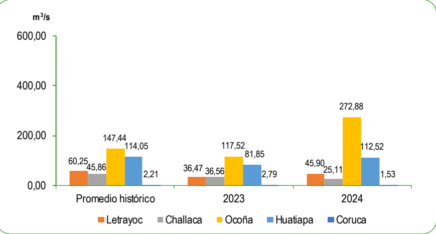
GRÁFICO N°43 PERÚ: CAUDAL PROMEDIO DE LOS RÍOS DE LA ZONA SUR DE LA VERTIENTE DEL PACÍFICO Abril 2023 – 2024 Metro cúbico por segundo (m³/s)
