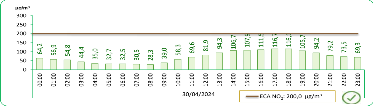
GRÁFICO N° 11 LIMA METROPOLITANA: VALOR DIARIO DEL DIÓXIDO DE NITRÓGENO (NO 2 ), EN LA ESTACIÓN DE MEDICIÓN DE PUENTE PIEDRA – ABRIL 2024
