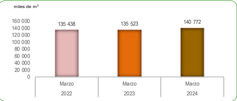
GRÁFICO N°38 PERÚ: PRODUCCIÓN NACIONAL DE AGUA POTABLE Marzo 2022 - 2024 Miles de metros cúbicos (Miles de m³)
