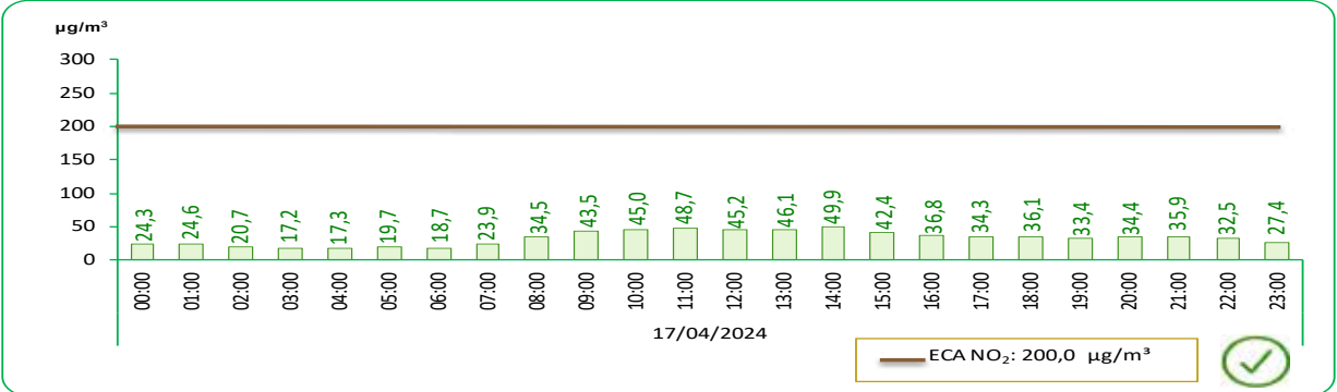
GRÁFICO N°13 LIMA METROPOLITANA: VALOR DIARIO DEL DIÓXIDO DE NITRÓGENO (NO 2 ), EN LA ESTACIÓN DE MEDICIÓN DE SAN BORJA – ABRIL 2024
