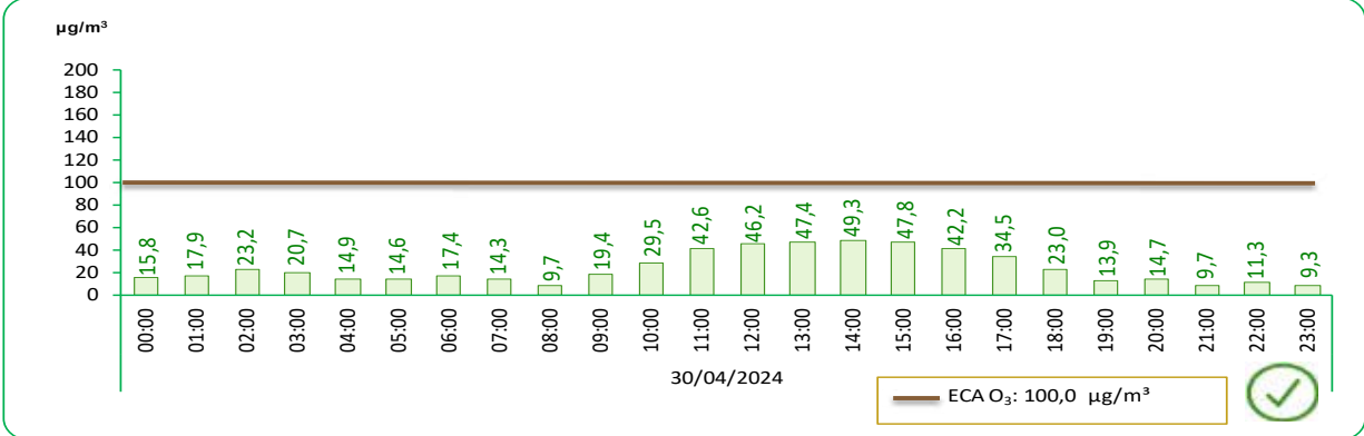
GRÁFICO N°23 LIMA METROPOLITANA: VALOR DIARIO DEL OZONO TROPOSFÉRICO (O 3 ), EN LA ESTACIÓN DE MEDICIÓN DE CAMPO DE MARTE – ABRIL 2024
