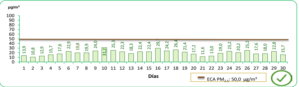
GRÁFICO N° 08 LIMA METROPOLITANA: CONCENTRACIÓN DIARIA DEL MATERIAL PARTICULADO INFERIOR A 2.5 MICRAS (PM 2.5 ), EN LA ESTACIÓN DE MEDICIÓN DE SANTA ANITA – ABRIL 2024
