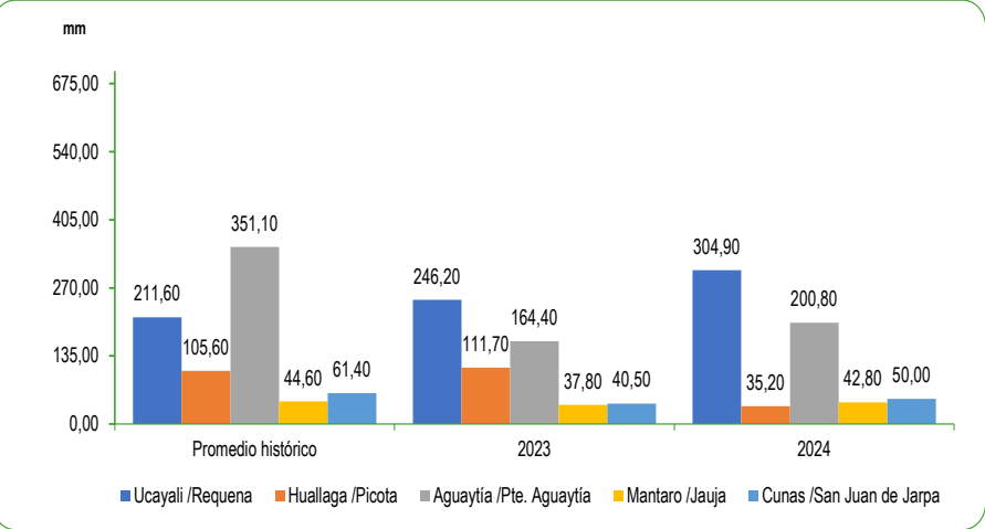
GRÁFICO N°51 PERÚ: PROMEDIO DE LAS PRECIPITACIONES EN LA ZONA CENTRO DE LA VERTIENTE DEL ATLÁNTICO Abril 2023 - 2024 Milímetros (mm)
