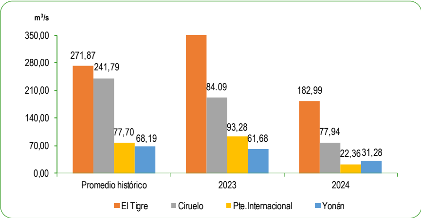
GRÁFICO N°41 PERÚ: CAUDAL PROMEDIO DE LOS RÍOS DE LA ZONA NORTE DE LA VERTIENTE DEL PACÍFICO Abril 2023 - 2024 Metro cúbico por segundo (m³/s)
