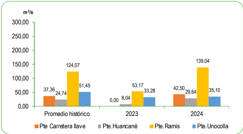
GRÁFICO N°46 PERÚ: CAUDAL PROMEDIO DE LOS RÍOS DE LA VERTIENTE DEL LAGO TITICACA Abril 2023 – 2024 Metro cúbico por segundo (m³/s)
