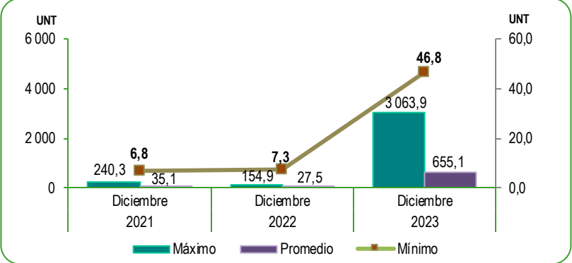
GRÁFICO N°37 LIMA METROPOLITANA: NIVELES DE TURBIEDAD EN EL RÍO RÍMAC Mes: Diciembre 2021 - 2023 Unidades Nefelométricas de Turbiedad (UNT)
