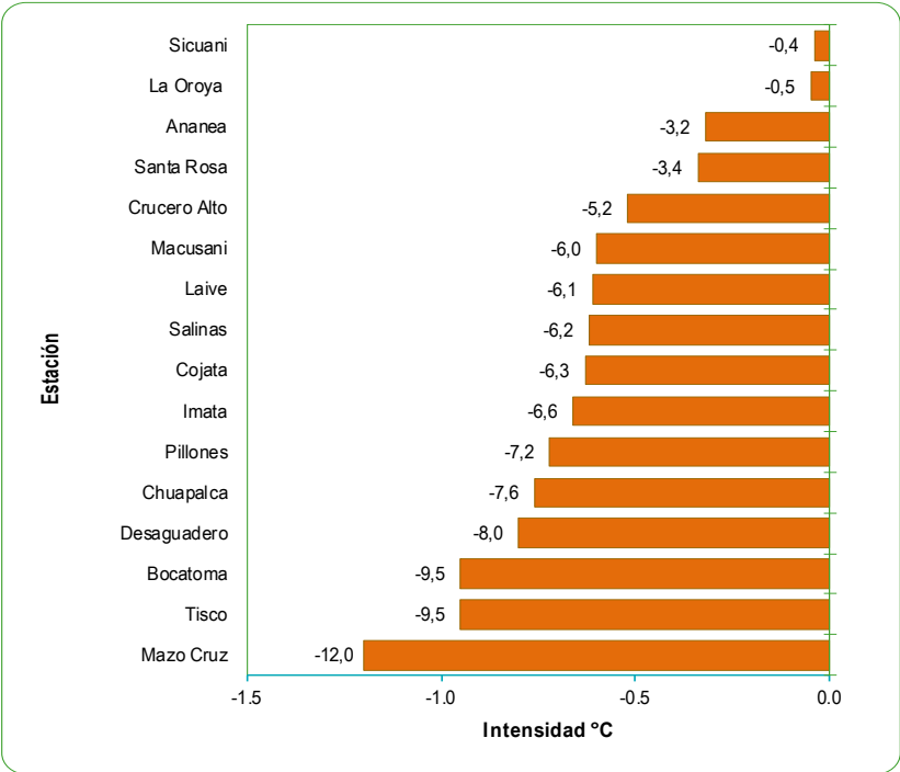
GRÁFICO N°56 PERÚ: MAYOR INTENSIDAD REGISTRADA DE LAS HELADAS METEOROLÓGICAS Abril 2024 Temperatura bajo cero grados
