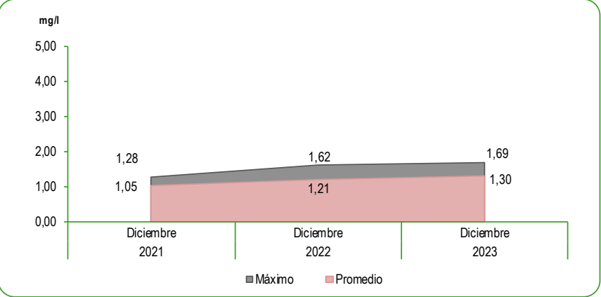
GRÁFICO N°34 LIMA METROPOLITANA: CONCENTRACIÓN DE MATERIA ORGÁNICA EXPRESADA COMO TOC EN LAS PLANTAS DE TRATAMIENTO 1 Y 2 DE SEDAPAL Diciembre 2021 - 2023 Miligramos por litro (mg/l)
