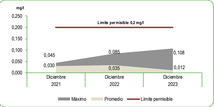
GRÁFICO N°32 LIMA METROPOLITANA: CONCENTRACIÓN DE ALUMINIO (Al) EN LAS PLANTAS DE TRATAMIENTO 1 Y 2 DE SEDAPAL Diciembre 2021 - 2023 Miligramos por litro (mg/l)
