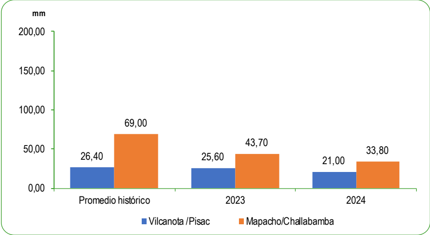
GRÁFICO N°52 PERÚ: PROMEDIO DE LAS PRECIPITACIONES EN LA ZONA SUR DE LA VERTIENTE DEL ATLÁNTICO Abril 2023 - 2024 Milímetros (mm)
