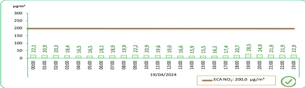
GRÁFICO N° 10 LIMA METROPOLITANA: VALOR DIARIO DEL DIÓXIDO DE NITRÓGENO (NO 2 ), EN LA ESTACIÓN DE MEDICIÓN DE SAN MARTIN DE PORRES – ABRIL 2024
