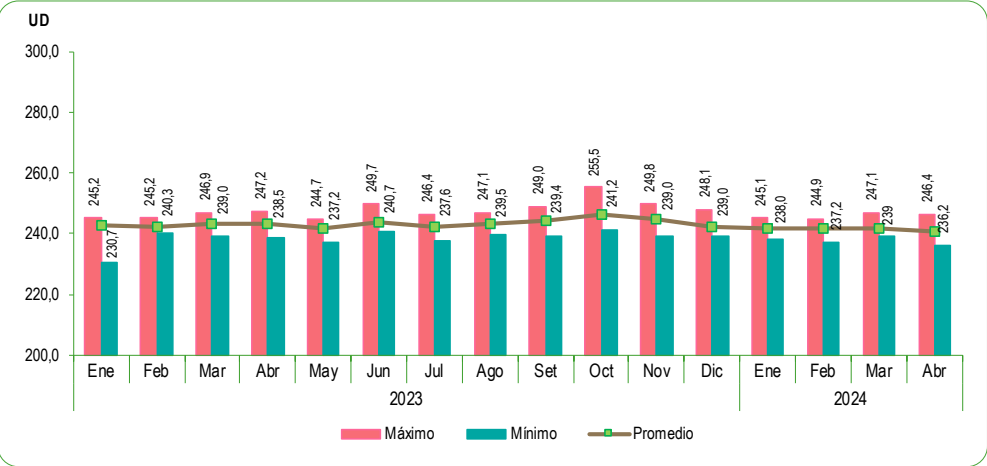
GRÁFICO N°24 PERÚ: VIGILANCIA DEL OZONO ATMOSFÉRICO EN LA ESTACIÓN VAG MARCAPOMACOA Abril 2023 – Abril 2024 Unidades Dobson (UD)
