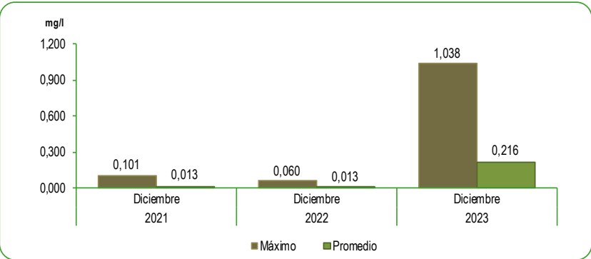
GRÁFICO N° 27 LIMA METROPOLITANA: CONCENTRACIÓN DE PLOMO (Pb) EN EL RÍO RÍMAC Diciembre 2021 - 2023 Miligramos por litro (mg/l)
