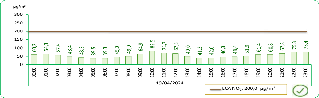
GRÁFICO N° 09 LIMA METROPOLITANA: VALOR DIARIO DEL DIÓXIDO DE NITRÓGENO (NO 2 ), EN LA ESTACIÓN DE MEDICIÓN DE CARABAYLLO – ABRIL 2024
