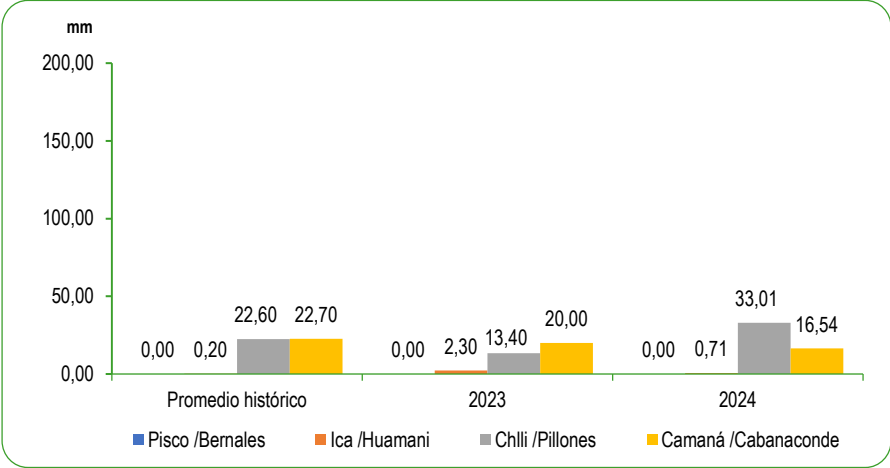
GRÁFICO N°49 PERÚ: PROMEDIO DE LAS PRECIPITACIONES EN LA ZONA SUR DE LA VERTIENTE DEL PACÍFICO Abril 2023 - 2024 Milímetros (mm)
