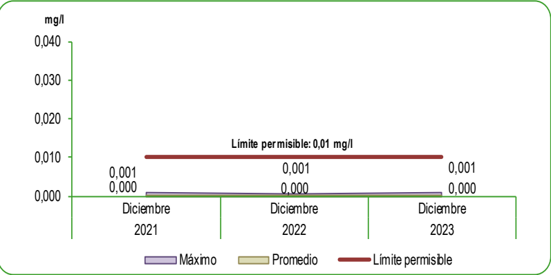
GRÁFICO N°28 LIMA METROPOLITANA: CONCENTRACIÓN DE PLOMO (Pb) EN LAS PLANTAS DE TRATAMIENTO 1 Y 2 DE SEDAPAL Diciembre 2021 - 2023 Miligramos por litro (mg/l)
