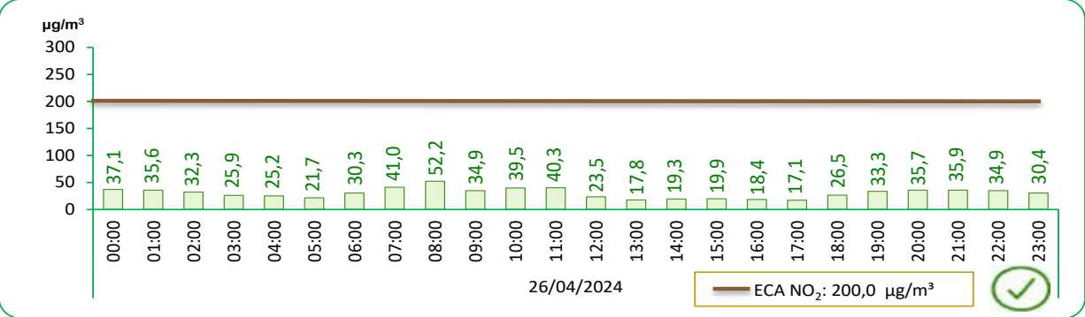
GRÁFICO N° 12 LIMA METROPOLITANA: VALOR DIARIO DEL DIÓXIDO DE NITRÓGENO (NO 2 ), EN LA ESTACIÓN DE MEDICIÓN DE CAMPO DE MARTE – ABRIL 2024
