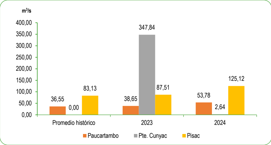
GRÁFICO N°45 PERÚ: CAUDAL PROMEDIO DE LOS RÍOS DE LA ZONA SUR DE LA VERTIENTE DEL ATLÁNTICO Abril 2023 – 2024 Metro cúbico por segundo (m³/s)
