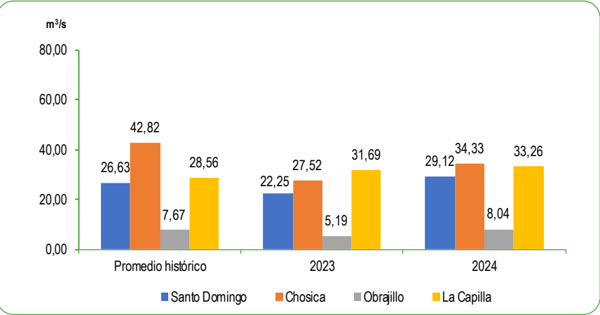
GRÁFICO N°42 PERÚ: CAUDAL PROMEDIO DE LOS RÍOS DE LA ZONA CENTRO DE LA VERTIENTE DEL PACÍFICO Abril 2023 – 2024 Metro cúbico por segundo (m³/s)
