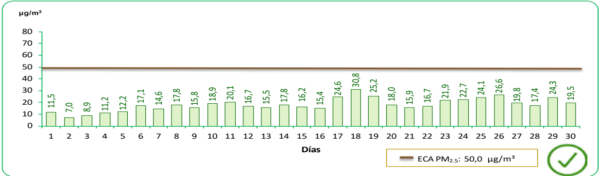
GRÁFICO N°07 LIMA METROPOLITANA: CONCENTRACIÓN DIARIA DEL MATERIAL PARTICULADO INFERIOR A 2.5 MICRAS (PM 2.5 ), EN LA ESTACIÓN DE MEDICIÓN DE CAMPO DE MARTE – ABRIL 2024
