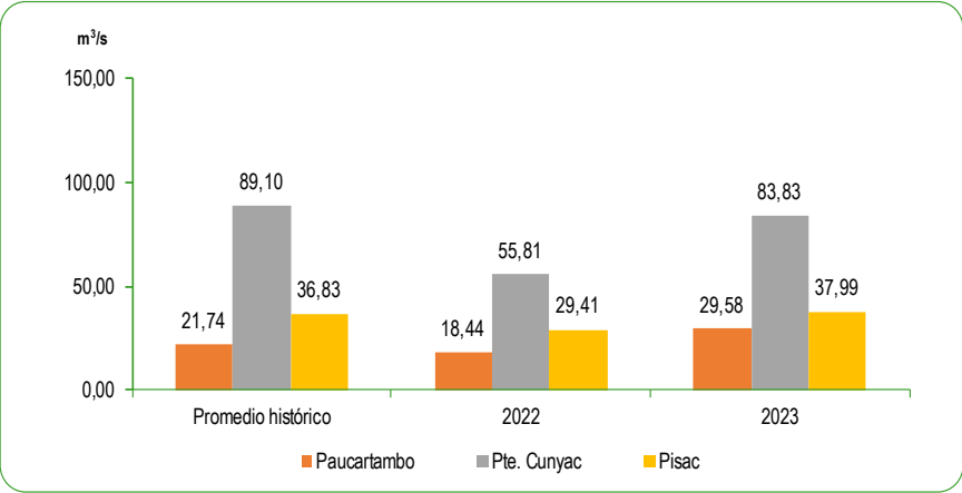
GRÁFICO N°55 PERÚ: CAUDAL PROMEDIO DE LOS RÍOS DE LA ZONA SUR DE LA VERTIENTE DEL ATLÁNTICO Mes: Noviembre 2022 - 2023 Metro cúbico por segundo (m³/s)
