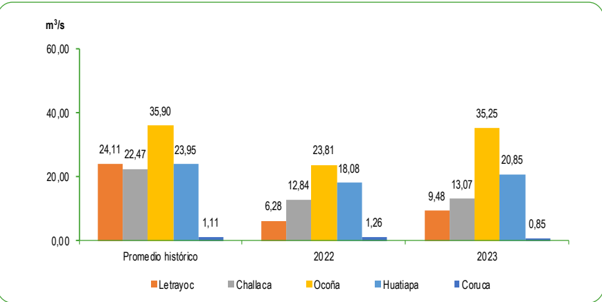
GRÁFICO N°53 PERÚ: CAUDAL PROMEDIO DE LOS RÍOS DE LA ZONA SUR DE LA VERTIENTE DEL PACÍFICO Mes: Noviembre 2022 – 2023 Metro cúbico por segundo (m³/s)
