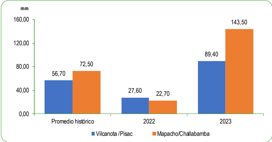
GRÁFICO N°62 PERÚ: PROMEDIO DE LAS PRECIPITACIONES EN LA ZONA SUR DE LA VERTIENTE DEL ATLÁNTICO Mes: Noviembre 2022 - 2023 Milímetros (mm)
