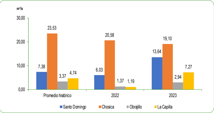
GRÁFICO N°52 PERÚ: CAUDAL PROMEDIO DE LOS RÍOS DE LA ZONA CENTRO DE LA VERTIENTE DEL PACÍFICO Mes: Noviembre 2022 – 2023 Metro cúbico por segundo (m³/s)
