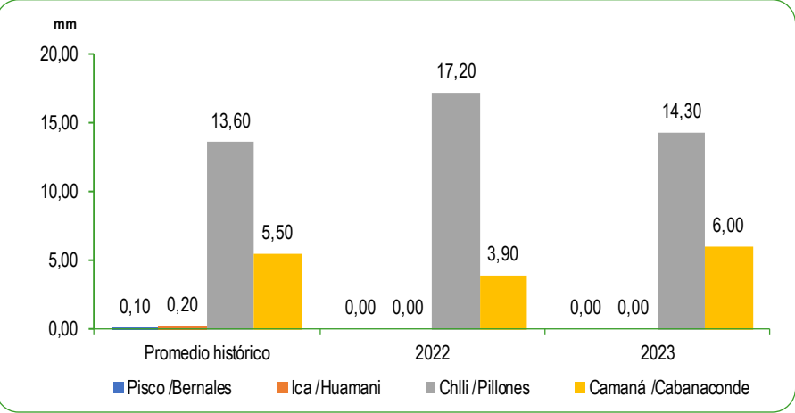
GRÁFICO N°59 PERÚ: PROMEDIO DE LAS PRECIPITACIONES EN LA ZONA SUR DE LA VERTIENTE DEL PACÍFICO Mes: Noviembre 2022 - 2023 Milímetros (mm)
