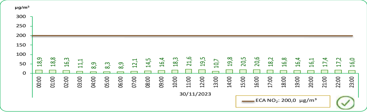
GRÁFICO N°27 LIMA METROPOLITANA: VALOR DIARIO DEL DIÓXIDO DE NITRÓGENO (NO 2 ), EN LA ESTACIÓN DE MEDICIÓN DE VILLA MARÍA DEL TRIUNFO – NOVIEMBRE 2023
