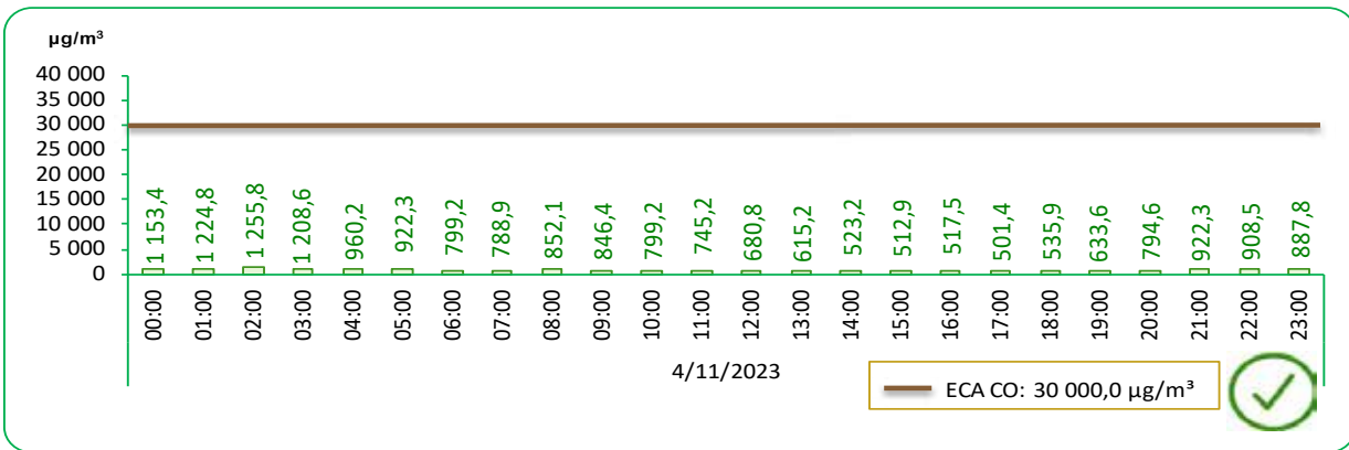
GRÁFICO N°28 LIMA METROPOLITANA: VALOR DIARIO DEL MONÓXIDO DE CARBONO (CO), EN LA ESTACIÓN DE MEDICIÓN DE CARABAYLLO – NOVIEMBRE 2023
