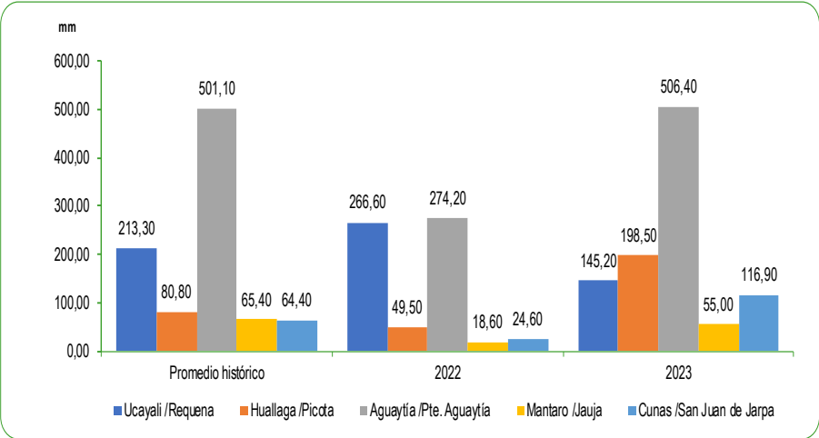
GRÁFICO N°61 PERÚ: PROMEDIO DE LAS PRECIPITACIONES EN LA ZONA CENTRO DE LA VERTIENTE DEL ATLÁNTICO Mes: Noviembre 2022 - 2023 Milímetros (mm)
