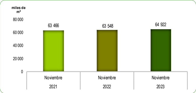
GRÁFICO N°49 LIMA METROPOLITANA: PRODUCCIÓN DE AGUA POTABLE Mes: Noviembre 2021 - 2023 Miles de metros cúbicos (Miles de m³)
