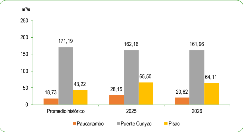
GRÁFICO N°64 PERÚ: CAUDAL PROMEDIO DE LOS RÍOS DE LA ZONA SUR DE LA VERTIENTE DEL ATLÁNTICO MAYO 2025 - 2026 Metro cúbico por segundo (m³/s)
