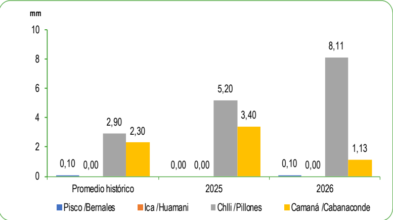
GRÁFICO N°68 PERÚ: PROMEDIO DE LAS PRECIPITACIONES EN LA ZONA SUR DE LA VERTIENTE DEL PACÍFICO MAYO 2025 - 2026 Milímetros (mm)
