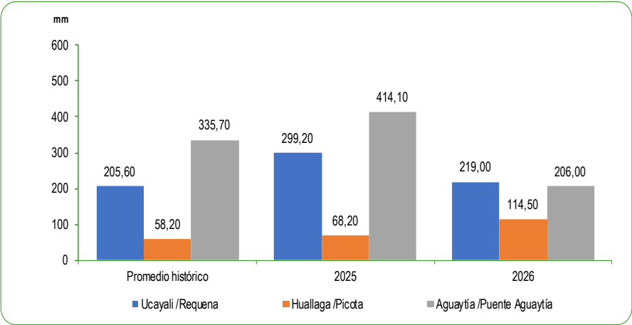
GRÁFICO N°70 PERÚ: PROMEDIO DE LAS PRECIPITACIONES EN LA ZONA CENTRO DE LA VERTIENTE DEL ATLÁNTICO MAYO 2025 - 2026 Milímetros (mm)
