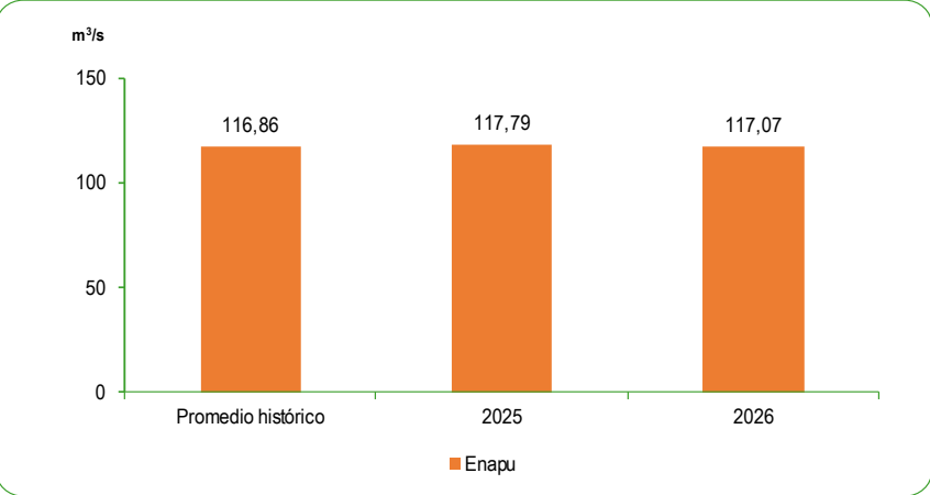
GRÁFICO N°62 PERÚ: CAUDAL PROMEDIO DE LOS RÍOS DE LA ZONA NORTE DE LA VERTIENTE DEL ATLÁNTICO MAYO 2025 - 2026 Metro cúbico por segundo (m³/s)
