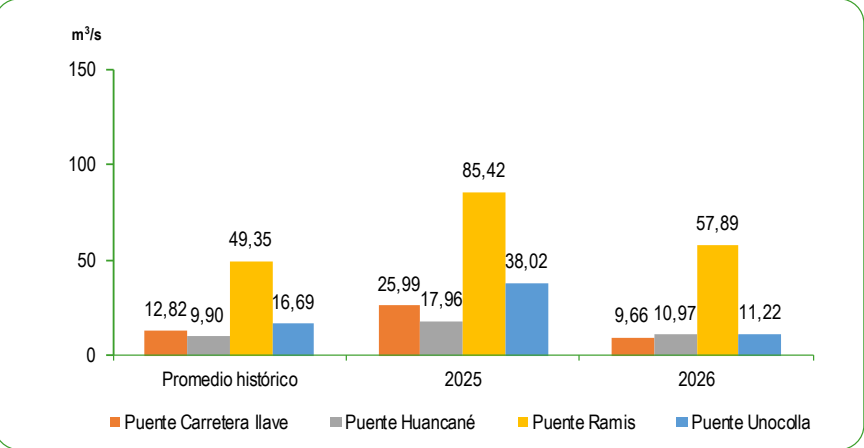
GRÁFICO N°65 PERÚ: CAUDAL PROMEDIO DE LOS RÍOS DE LA VERTIENTE DEL LAGO TITICACA MAYO 2025 – 2026 Metro cúbico por segundo (m³/s)
