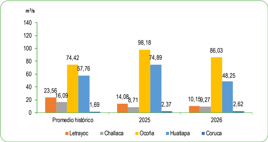
GRÁFICO N°61 PERÚ: CAUDAL PROMEDIO DE LOS RÍOS DE LA ZONA SUR DE LA VERTIENTE DEL PACÍFICO MAYO 2024 – 2025 Metro cúbico por segundo (m³/s)
