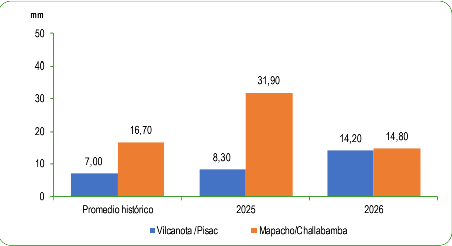
GRÁFICO N°71 PERÚ: PROMEDIO DE LAS PRECIPITACIONES EN LA ZONA SUR DE LA VERTIENTE DEL ATLÁNTICO MAYO 2025 - 2026 Milímetros (mm)
