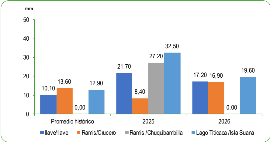
GRÁFICO N°72 PERÚ: PROMEDIO DE LAS PRECIPITACIONES EN LA VERTIENTE DEL LAGO TITICACA MAYO 2025 - 2026 Milímetros (mm)
