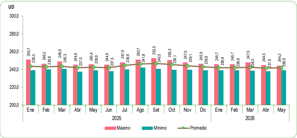
GRÁFICO N°42 PERÚ: VIGILANCIA DEL OZONO ATMOSFÉRICO EN LA ESTACIÓN VAG MARCAPOMACOA MAYO 2026 – MAYO 2025 Unidades Dobson (UD)
