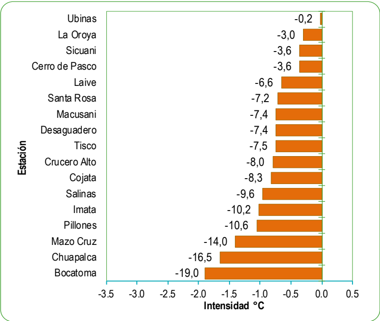
GRÁFICO N°75 PERÚ: MAYOR INTENSIDAD REGISTRADA DE LAS HELADAS METEOROLÓGICAS MAYO 2026 Temperatura bajo cero grados
