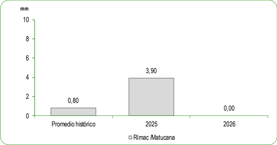
GRÁFICO N°67 PERÚ: PROMEDIO DE LAS PRECIPITACIONES EN LA ZONA CENTRO DE LA VERTIENTE DEL PACÍFICO MAYO 2025 - 2026 Milímetros (mm)
