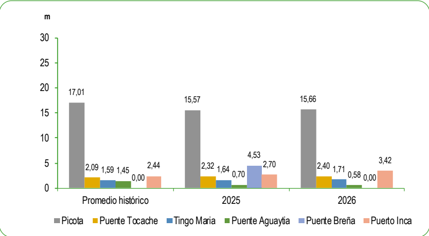
GRÁFICO N°63 PERÚ: CAUDAL PROMEDIO DE LOS RÍOS DE LA ZONA CENTRO DE LA VERTIENTE DEL ATLÁNTICO MAYO 2025 - 2026 Metro (m)
