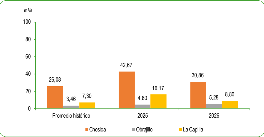
GRÁFICO N°60 PERÚ: CAUDAL PROMEDIO DE LOS RÍOS DE LA ZONA CENTRO DE LA VERTIENTE DEL PACÍFICO MAYO 2025 - 2026 Metro cúbico por segundo (m³/s)
