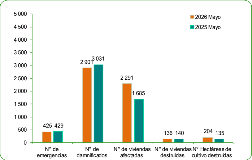
GRÁFICO N°73 PERÚ: NÚMERO DE EMERGENCIAS Y DAÑOS PRODUCIDOS A NIVEL NACIONAL MAYO 2026 / MAYO 2025 Número (N°)
