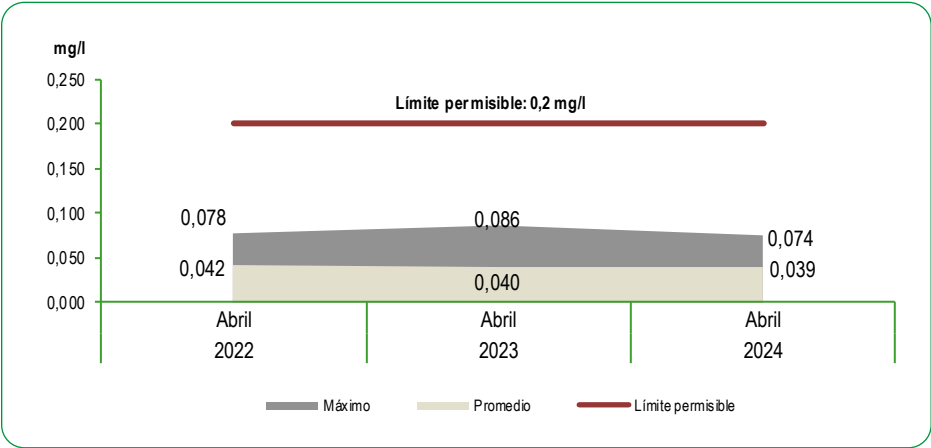
GRÁFICO N°38 LIMA METROPOLITANA: CONCENTRACIÓN DE ALUMINIO (Al) EN LAS PLANTAS DE TRATAMIENTO 1 Y 2 DE SEDAPAL Abril 2022 - 2024 Miligramos por litro (mg/l)
