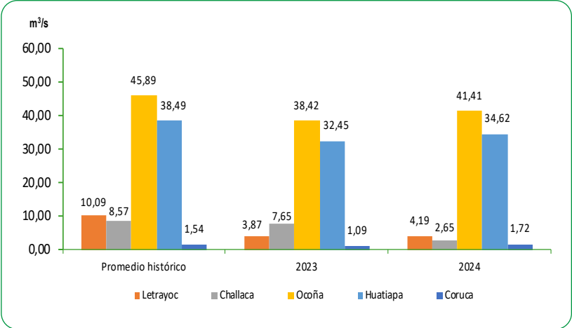
GRÁFICO N°49 PERÚ: CAUDAL PROMEDIO DE LOS RÍOS DE LA ZONA SUR DE LA VERTIENTE DEL PACÍFICO Julio 2023 – 2024 Metro cúbico por segundo (m³/s)
