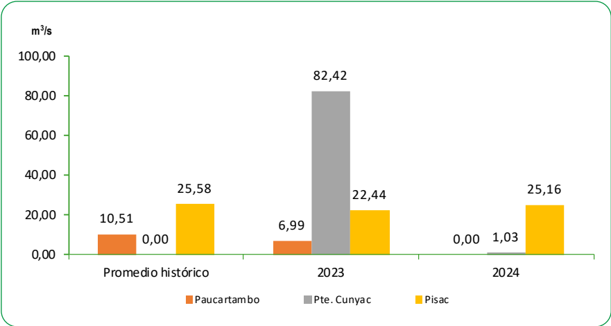
GRÁFICO N° 52 PERÚ: CAUDAL PROMEDIO DE LOS RÍOS DE LA ZONA SUR DE LA VERTIENTE DEL ATLÁNTICO Julio 2023 – 2024 Metro cúbico por segundo (m³/s)
