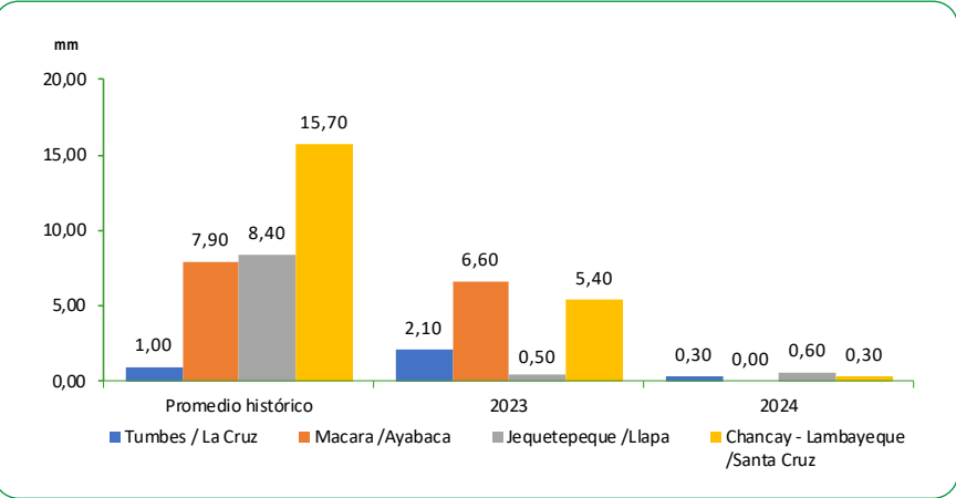
GRÁFICO N°54 PERÚ: PROMEDIO DE LAS PRECIPITACIONES EN LA ZONA NORTE DE LA VERTIENTE DEL PACÍFICO Julio 2023 - 2024 Milímetros (mm)
