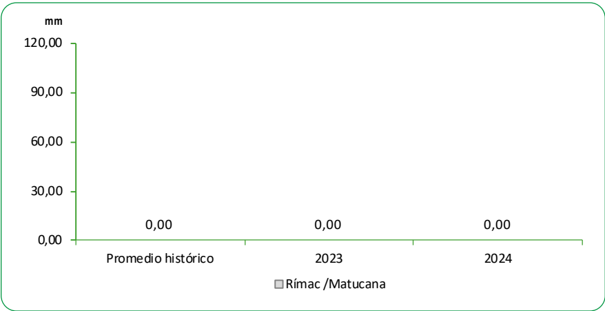
GRÁFICO N°55 PERÚ: PROMEDIO DE LAS PRECIPITACIONES EN LA ZONA CENTRO DE LA VERTIENTE DEL PACÍFICO Julio 2023 - 2024 Milímetros (mm)
