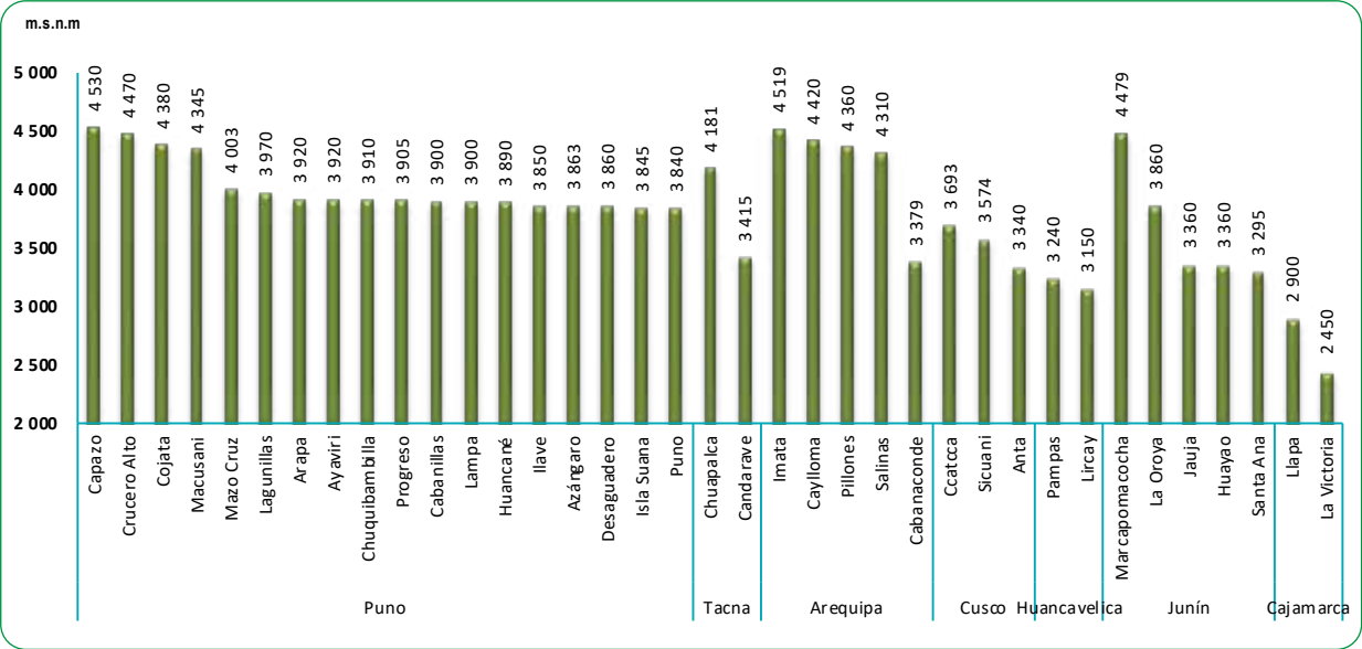
GRÁFICO N°64 PERÚ: ALTITUD DE LAS ESTACIONES METEOROLÓGICAS Metros sobre el nivel del mar
