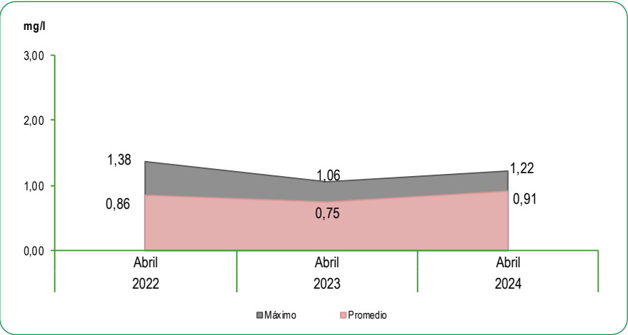
GRÁFICO N°40 LIMA METROPOLITANA: CONCENTRACIÓN DE MATERIA ORGÁNICA EXPRESADA COMO TOC EN LAS PLANTAS DE TRATAMIENTO 1 Y 2 DE SEDAPAL Abril 2022 - 2024 Miligramos por litro (mg/l)
