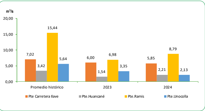
GRÁFICO N°53 PERÚ: CAUDAL PROMEDIO DE LOS RÍOS DE LA VERTIENTE DEL LAGO TITICACA Julio 2023 – 2024 Metro cúbico por segundo (m³/s)
