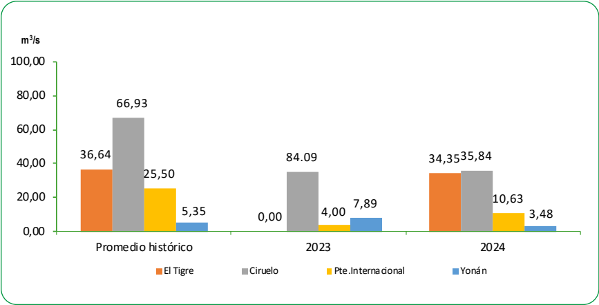
GRÁFICO N°47 PERÚ: CAUDAL PROMEDIO DE LOS RÍOS DE LA ZONA NORTE DE LA VERTIENTE DEL PACÍFICO Julio 2023 - 2024 Metro cúbico por segundo (m³/s)
