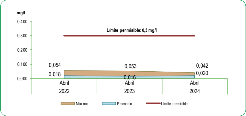
GRÁFICO N°32 LIMA METROPOLITANA: CONCENTRACIÓN DE HIERRO (Fe) EN LAS PLANTAS DE TRATAMIENTO 1 Y 2 DE SEDAPAL Abril 2022 - 2024 Miligramos por litro (mg/l)
