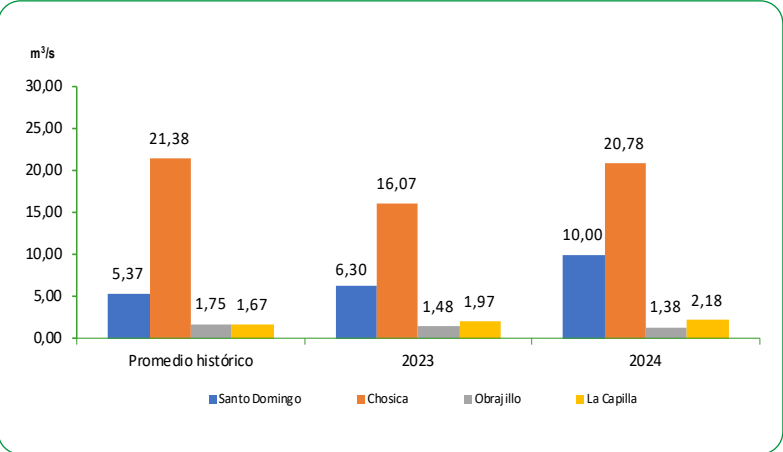
GRÁFICO N° 48 PERÚ: CAUDAL PROMEDIO DE LOS RÍOS DE LA ZONA CENTRO DE LA VERTIENTE DEL PACÍFICO Julio 2023 – 2024 Metro cúbico por segundo (m³/s)
