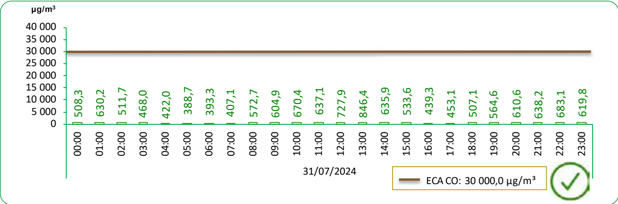
ZONA LIMA CENTRO GRÁFICO N°28 LIMA METROPOLITANA: VALOR DIARIO DEL MONÓXIDO DE CARBONO (CO), EN LA ESTACIÓN DE MEDICIÓN DE CAMPO DE MARTE – JULIO 2024
