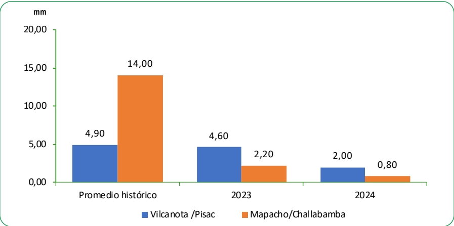
GRÁFICO N°59 PERÚ: PROMEDIO DE LAS PRECIPITACIONES EN LA ZONA SUR DE LA VERTIENTE DEL ATLÁNTICO Julio 2023 - 2024 Milímetros (mm)
