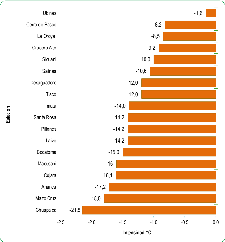
GRÁFICO N°63 PERÚ: MAYOR INTENSIDAD REGISTRADA DE LAS HELADAS METEOROLÓGICAS Julio 2024 Temperatura bajo cero grados
