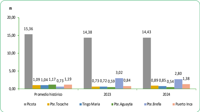
GRÁFICO N°51 PERÚ: CAUDAL PROMEDIO DE LOS RÍOS DE LA ZONA CENTRO DE LA VERTIENTE DEL ATLÁNTICO Julio 2023 – 2024 Metro (m)
