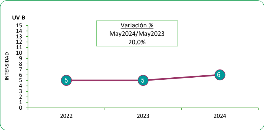
GRÁFICO N°02: CIUDAD DE LIMA: ÍNDICE DE RADIACIÓN ULTRAVIOLETA, SEGÚN MÁXIMO MENSUAL Mayo 2022 a 2024 Índice de radiación ultravioleta (IUV)
