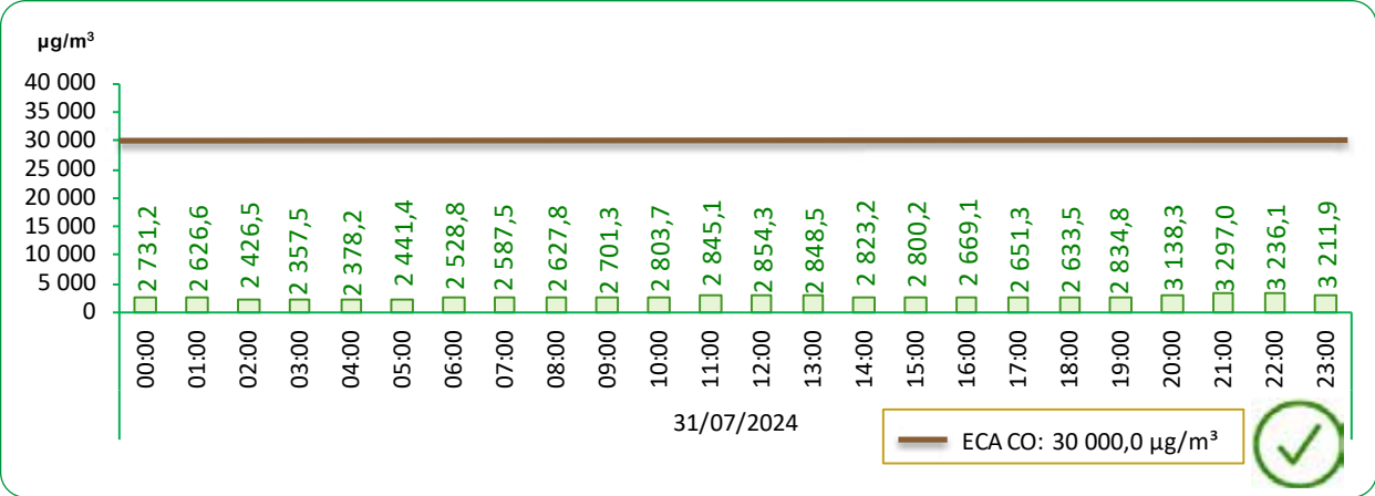
GRÁFICO N°27 LIMA METROPOLITANA: VALOR DIARIO DEL MONÓXIDO DE CARBONO (CO), EN LA ESTACIÓN DE MEDICIÓN DE PUENTE PIEDRA – JULIO 2024
