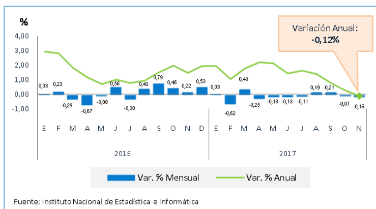
VARIACIÓN PORCENTUAL MENSUAL Y ANUAL DEL ÍNDICE DE PRECIOS AL POR MAYOR: ENERO 2016 - NOVIEMBRE 2017
