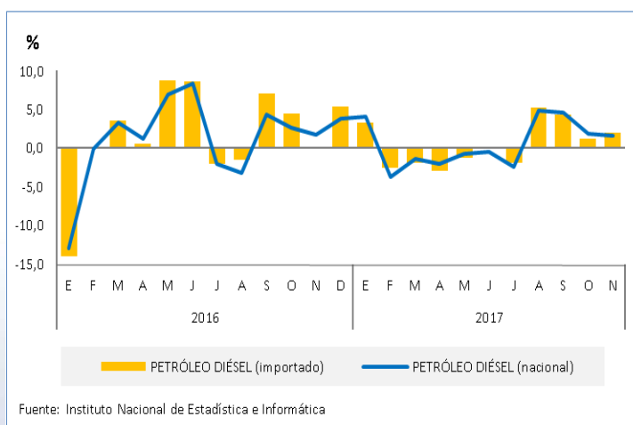
VARIACIÓN PORCENTUAL MENSUAL DE PRECIOS AL POR MAYOR DEL PETRÓLEO DIÉSEL NACIONAL E IMPORTADO: ENERO 2016 - NOVIEMBRE 2017
