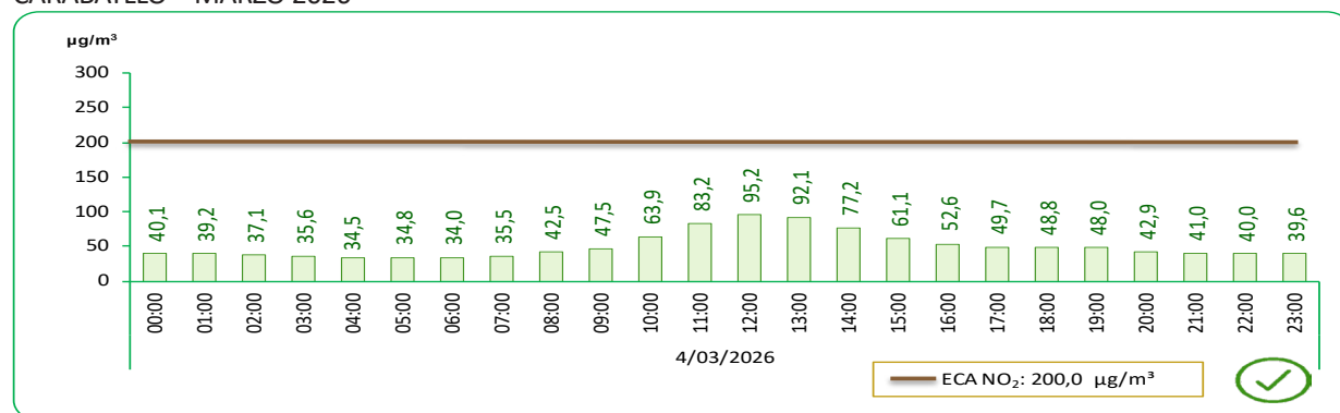
LIMA METROPOLITANA: VALOR DIARIO DEL DIÓXIDO DE NITRÓGENO (NO 2 ), EN LA ESTACIÓN DE MEDICIÓN DE CARABAYLLO – MARZO 2026
