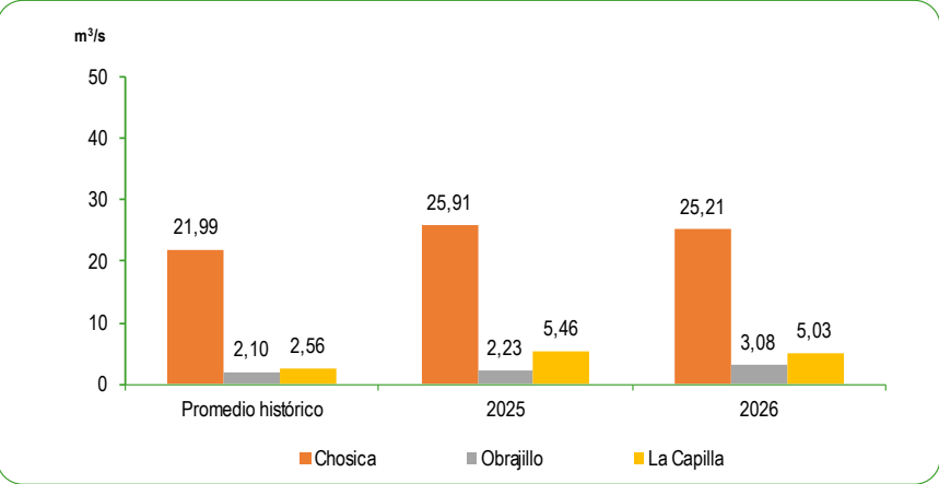
GRÁFICO N°62 PERÚ: CAUDAL PROMEDIO DE LOS RÍOS DE LA ZONA CENTRO DE LA VERTIENTE DEL PACÍFICO JUNIO 2025 - 2026 Metro cúbico por segundo (m³/s)
