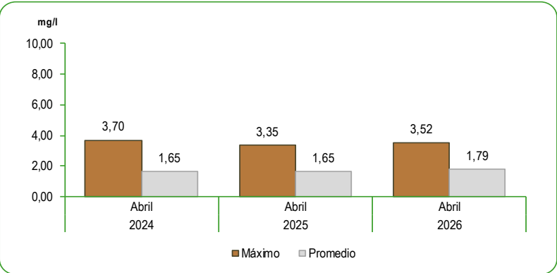
GRÁFICO N°53 LIMA METROPOLITANA: CONCENTRACIÓN DE MATERIA ORGÁNICA EXPRESADA COMO TOC EN EL RÍO RÍMAC Mes: Abril 2024 - 2026 Miligramos por litro (mg/l)
