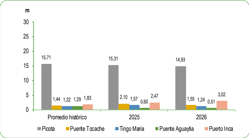
GRÁFICO N°65 PERÚ: CAUDAL PROMEDIO DE LOS RÍOS DE LA ZONA CENTRO DE LA VERTIENTE DEL ATLÁNTICO JUNIO 2025 - 2026 Metro (m)
