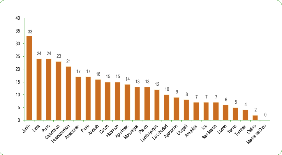
GRÁFICO N°76 PERÚ: NÚMERO DE EMERGENCIAS OCURRIDAS, SEGÚN DEPARTAMENTO JUNIO 2026 Número (N°)
