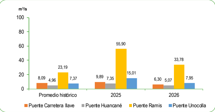
GRÁFICO N°67 PERÚ: CAUDAL PROMEDIO DE LOS RÍOS DE LA VERTIENTE DEL LAGO TITICACA JUNIO 2025 – 2026 Metro cúbico por segundo (m³/s)
