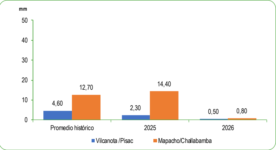
GRÁFICO N°73 PERÚ: PROMEDIO DE LAS PRECIPITACIONES EN LA ZONA SUR DE LA VERTIENTE DEL ATLÁNTICO JUNIO 2025 - 2026 Milímetros (mm)
