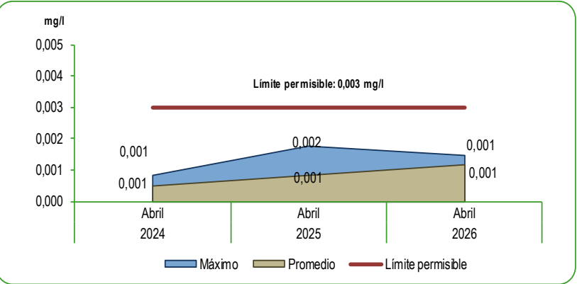
GRÁFICO N°50 LIMA METROPOLITANA: CONCENTRACIÓN DE CADMIO (Cd) EN LAS PLANTAS DE TRATAMIENTO 1 Y 2 DE SEDAPAL Mes: Abril 2024 - 2026 Miligramos por litro (mg/l)
