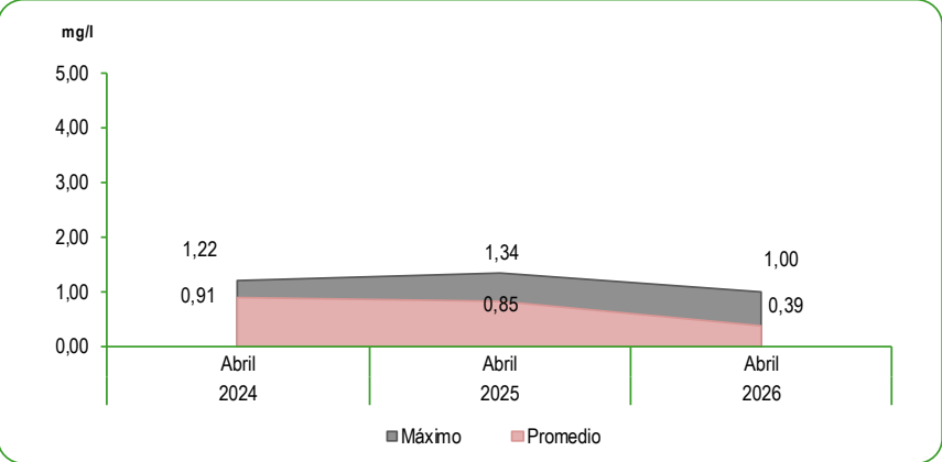
GRÁFICO N°54 LIMA METROPOLITANA: CONCENTRACIÓN DE MATERIA ORGÁNICA EXPRESADA COMO TOC EN LAS PLANTAS DE TRATAMIENTO 1 Y 2 DE SEDAPAL Mes: Abril 2024 - 2026 Miligramos por litro (mg/l)
