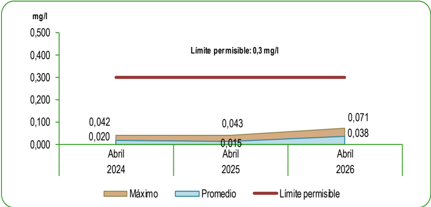
GRÁFICO N°46 LIMA METROPOLITANA: CONCENTRACIÓN DE HIERRO (Fe) EN LAS PLANTAS DE TRATAMIENTO 1 Y 2 DE SEDAPAL Mes: Abril 2024 - 2026 Miligramos por litro (mg/l)
