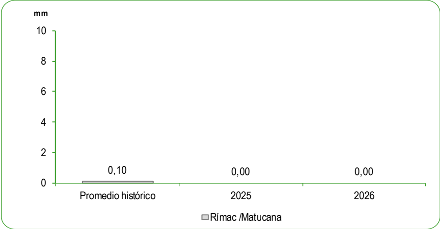
GRÁFICO N°69 PERÚ: PROMEDIO DE LAS PRECIPITACIONES EN LA ZONA CENTRO DE LA VERTIENTE DEL PACÍFICO JUNIO 2025 - 2026 Milímetros (mm)
