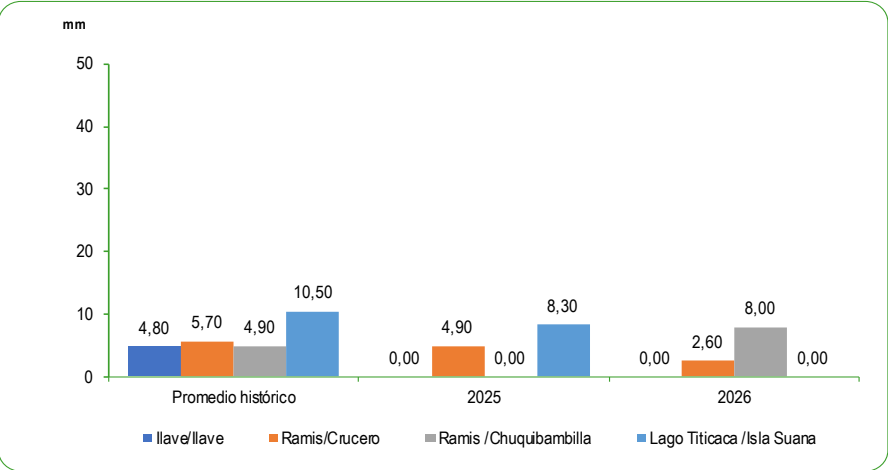
GRÁFICO N°74 PERÚ: PROMEDIO DE LAS PRECIPITACIONES EN LA VERTIENTE DEL LAGO TITICACA JUNIO 2025 - 2026 Milímetros (mm)
