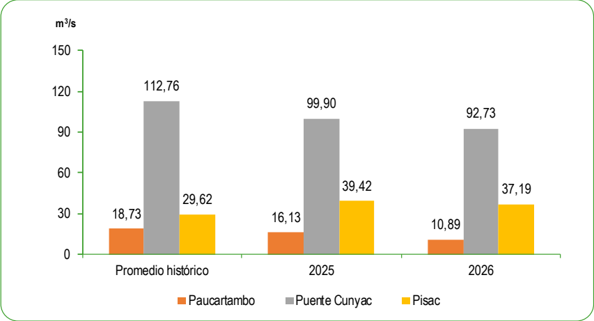
GRÁFICO N°66 PERÚ: CAUDAL PROMEDIO DE LOS RÍOS DE LA ZONA SUR DE LA VERTIENTE DEL ATLÁNTICO JUNIO 2025 - 2026 Metro cúbico por segundo (m³/s)
