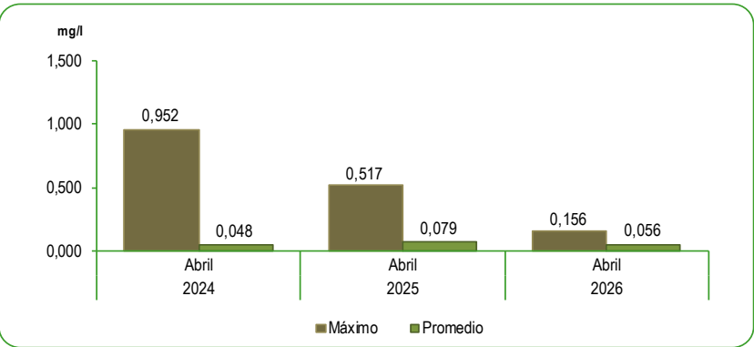
GRÁFICO N°47 LIMA METROPOLITANA: CONCENTRACIÓN DE PLOMO (Pb) EN EL RÍO RÍMAC Mes: Abril 2024 - 2026 Miligramos por litro (mg/l)
