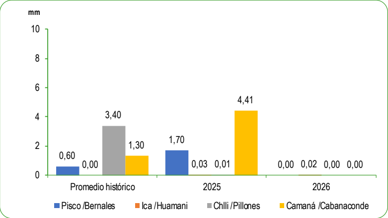
GRÁFICO N°70 PERÚ: PROMEDIO DE LAS PRECIPITACIONES EN LA ZONA SUR DE LA VERTIENTE DEL PACÍFICO JUNIO 2025 - 2026 Milímetros (mm)
