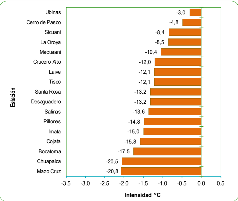
GRÁFICO N°77 PERÚ: MAYOR INTENSIDAD REGISTRADA DE LAS HELADAS METEOROLÓGICAS JUNIO 2026 Temperatura bajo cero grados
