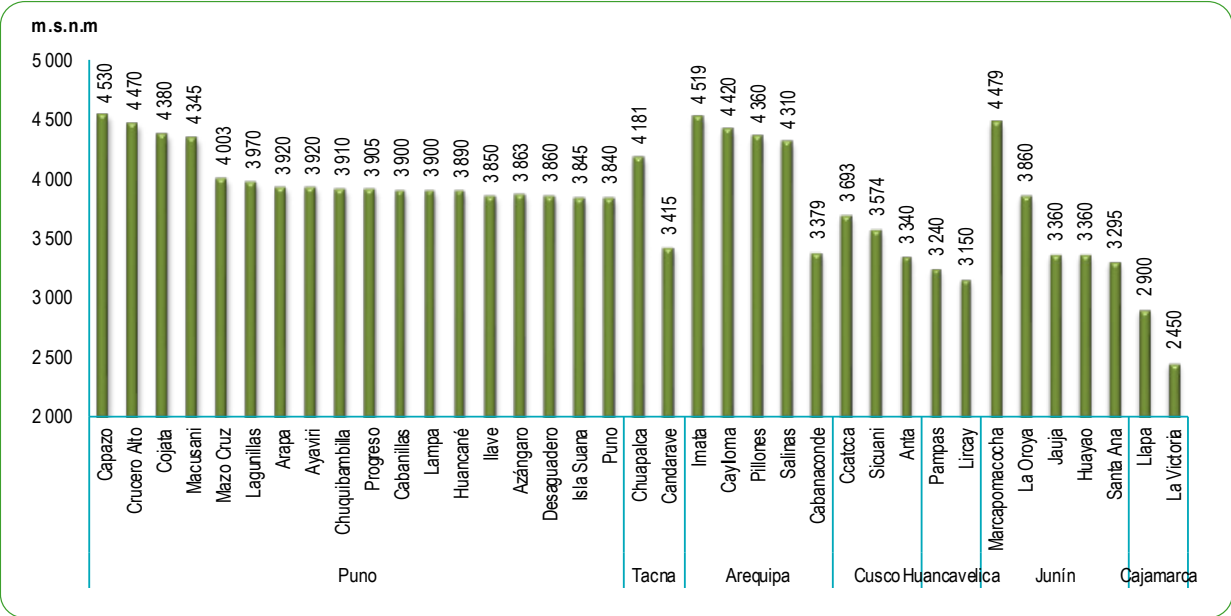
GRÁFICO N°78 PERÚ: ALTITUD DE LAS ESTACIONES METEOROLÓGICAS Metros sobre el nivel del mar
