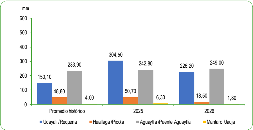
GRÁFICO N°72 PERÚ: PROMEDIO DE LAS PRECIPITACIONES EN LA ZONA CENTRO DE LA VERTIENTE DEL ATLÁNTICO JUNIO 2025 - 2026 Milímetros (mm)
