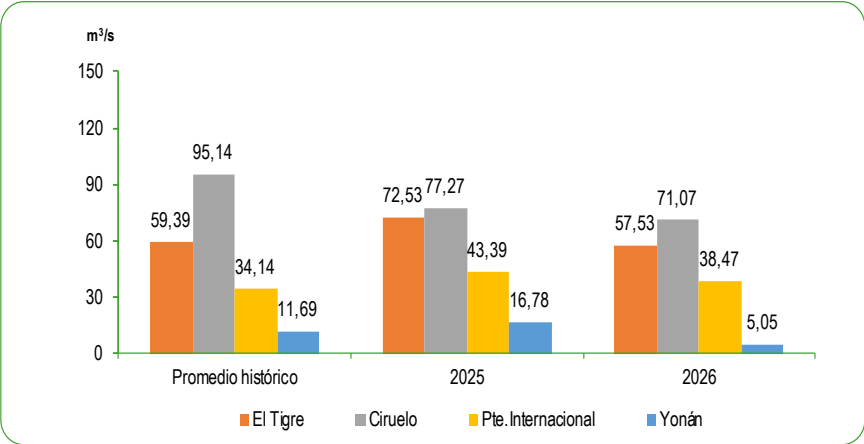
GRÁFICO N°61 PERÚ: CAUDAL PROMEDIO DE LOS RÍOS DE LA ZONA NORTE DE LA VERTIENTE DEL PACÍFICO JUNIO 2025 - 2026 Metro cúbico por segundo (m³/s)
