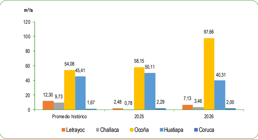
GRÁFICO N°63 PERÚ: CAUDAL PROMEDIO DE LOS RÍOS DE LA ZONA SUR DE LA VERTIENTE DEL PACÍFICO JUNIO 2024 – 2025 Metro cúbico por segundo (m³/s)
