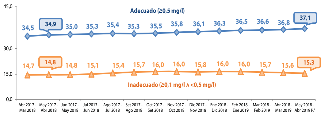
Gráfico N° 10 Perú: Población que consume agua proveniente de red pública, por niveles de cloro Año móvil: Mayo 2018 - Abril 2019 (Porcentaje)
