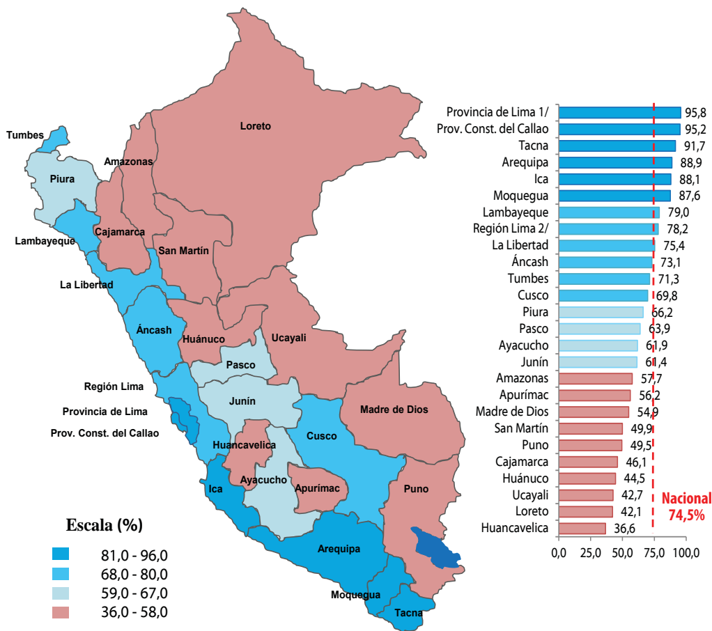
Gráfico N° 59 Perú: Población con acceso a red pública de alcantarillado, según departamento, 2018 (Porcentaje)
