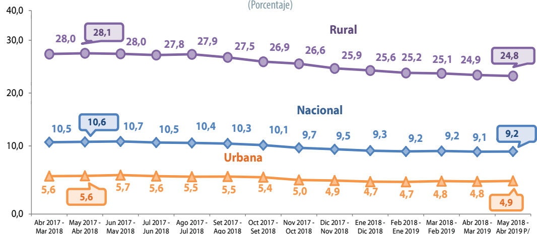
Gráfico N° 05 Perú: Población sin acceso a agua por red pública, por área de residencia Año móvil: Mayo 2018 - Abril 2019 (Porcentaje)
