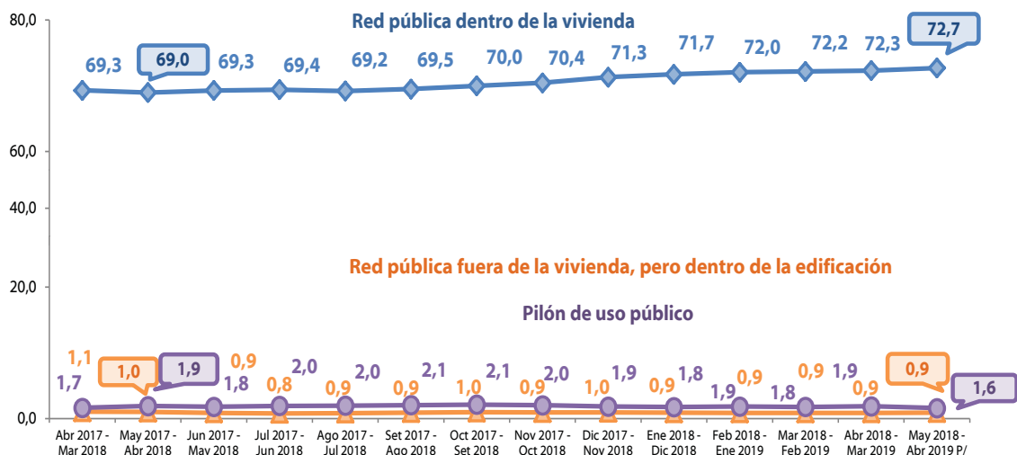
Gráfico N° 04 Perú-Rural: Población que consume agua proveniente de red pública, por tipo de conexión Año móvil: Mayo 2018 - Abril 2019 (Porcentaje)
