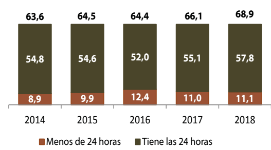
Gráfico N° 47 Perú - Rural: Población que consume agua proveniente de red pública las 24 horas del día, 2014 - 2018 (Porcentaje)
