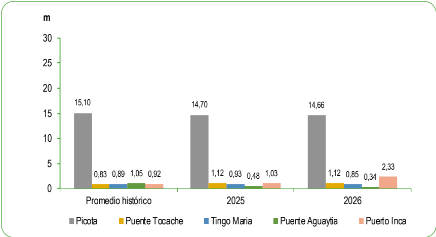
GRÁFICO N°62 PERÚ: CAUDAL PROMEDIO DE LOS RÍOS DE LA ZONA CENTRO DE LA VERTIENTE DEL ATLÁNTICO AGOSTO 2025 - 2026 Metro (m)
