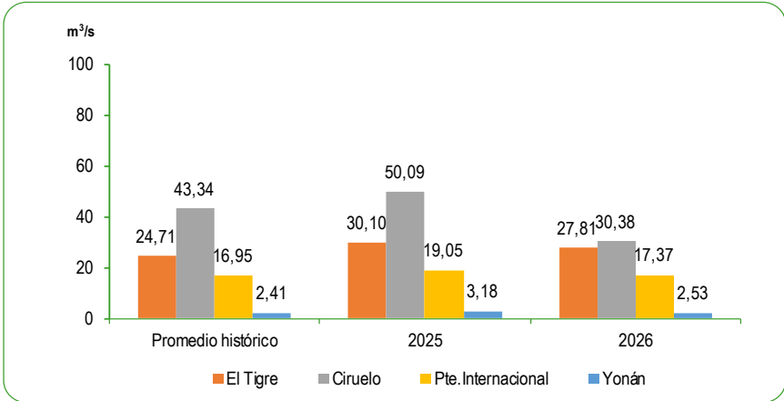
GRÁFICO N°58 PERÚ: CAUDAL PROMEDIO DE LOS RÍOS DE LA ZONA NORTE DE LA VERTIENTE DEL PACÍFICO AGOSTO 2025 - 2026 Metro cúbico por segundo (m³/s)
