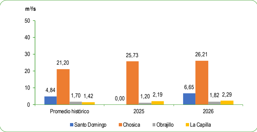
GRÁFICO N°59 PERÚ: CAUDAL PROMEDIO DE LOS RÍOS DE LA ZONA CENTRO DE LA VERTIENTE DEL PACÍFICO AGOSTO 2025 - 2026 Metro cúbico por segundo (m³/s)
