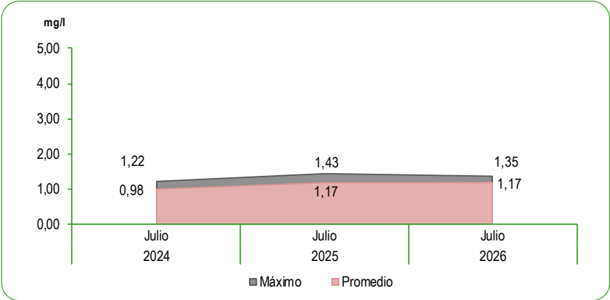
GRÁFICO N°51 LIMA METROPOLITANA: CONCENTRACIÓN DE MATERIA ORGÁNICA EXPRESADA COMO TOC EN LAS PLANTAS DE TRATAMIENTO 1 Y 2 DE SEDAPAL Mes: Julio 2024 - 2026 Miligramos por litro (mg/l)
