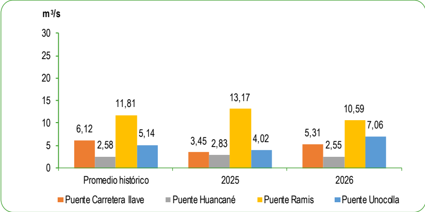
GRÁFICO N°64 PERÚ: CAUDAL PROMEDIO DE LOS RÍOS DE LA VERTIENTE DEL LAGO TITICACA AGOSTO 2025 – 2026 Metro cúbico por segundo (m³/s)
