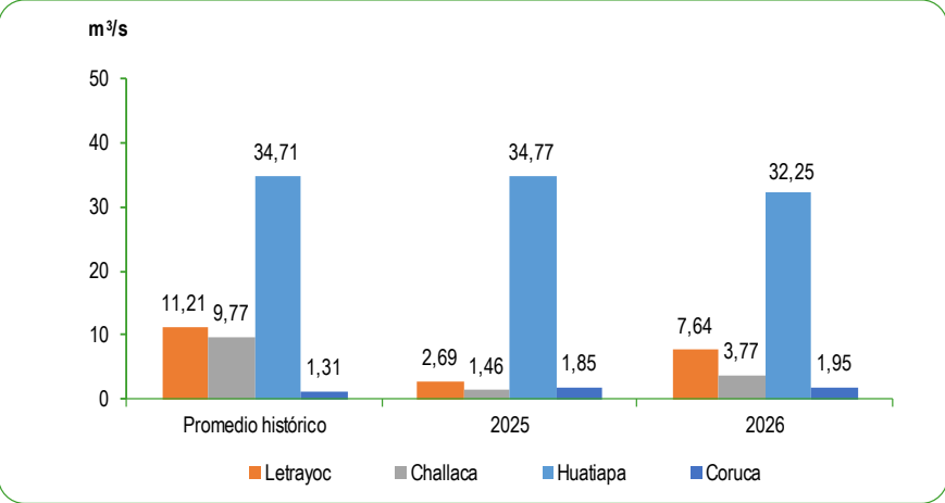
GRÁFICO N°60 PERÚ: CAUDAL PROMEDIO DE LOS RÍOS DE LA ZONA SUR DE LA VERTIENTE DEL PACÍFICO AGOSTO 2025 - 2026 Metro cúbico por segundo (m³/s)
