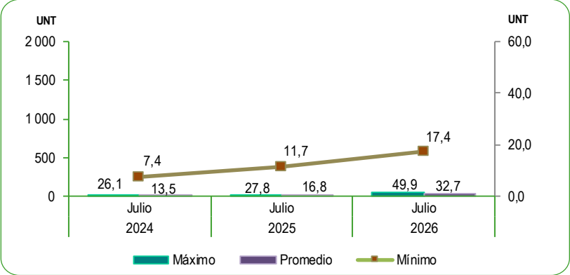
GRÁFICO N°54 LIMA METROPOLITANA: NIVELES DE TURBIEDAD EN EL RÍO RÍMAC Mes: Julio 2024 - 2026 Unidades Nefelométricas de Turbiedad (UNT)
