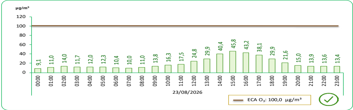
GRÁFICO N°32 LIMA METROPOLITANA: VALOR DIARIO DEL OZONO TROPOSFÉRICO (O 3 ), EN LA ESTACIÓN DE MEDICIÓN DE CARABAYLLO – AGOSTO 2026
