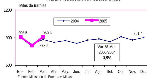
Piura: Producción de Petróleo Crudo
