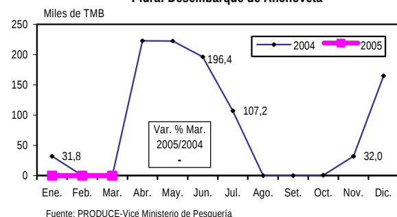
Piura: Desembarque de Anchoveta
