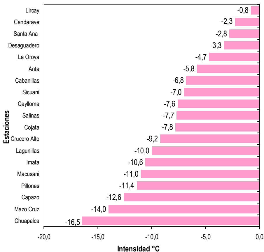
Gráfico N° 45 Perú: Intensidad de las heladas meteorológicas, mayo 2012 (Temperatura bajo cero)
