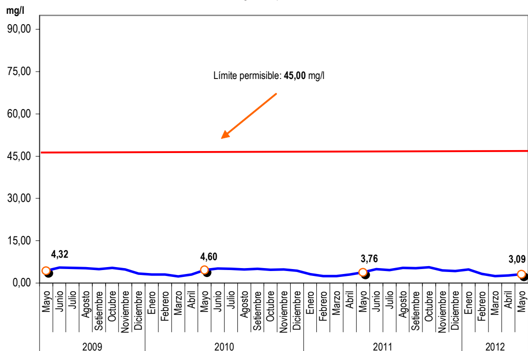
Gráfico N° 30 Lima Metropolitana: Concentración promedio mensual de nitratos en las plantas de tratamiento 1 y 2 de SEDAPAL, 2009-2012 Miligramos por litro
