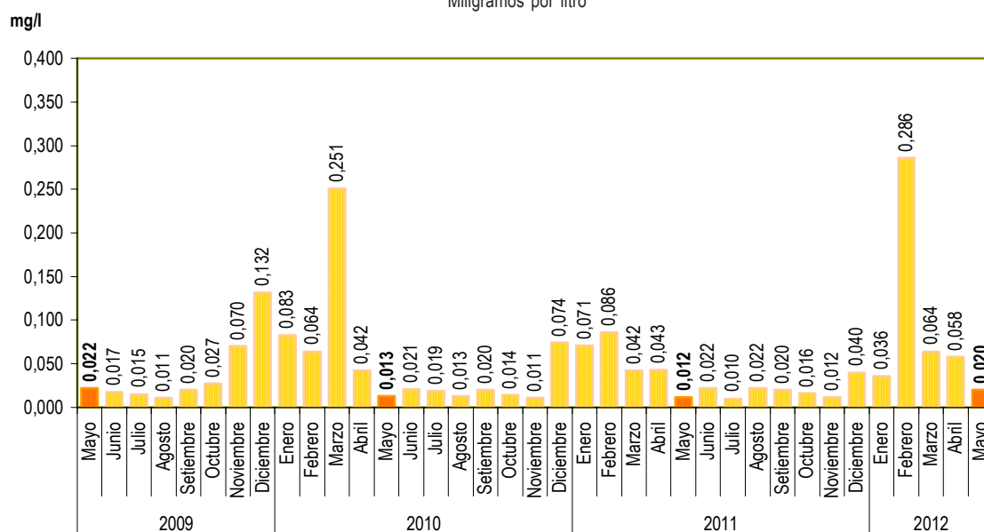
Gráfico N° 12 Lima Metropolitana: Concentración promedio mensual de plomo (Pb) en el río Rímac, 2009-2012 Miligramos por litro
