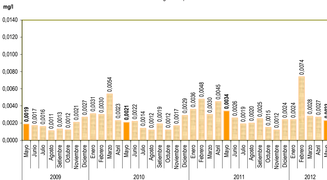
Gráfico N° 16 Lima Metropolitana: Concentración promedio mensual de cadmio (Cd) en el río Rímac, 2009-2012 Miligramos por litro
