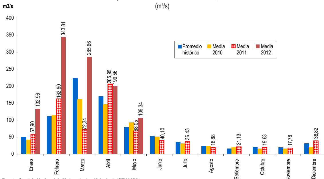
Gráfico N° 37 Perú: Caudal promedio de los ríos de la zona norte, 2010-2012 (m 3 /s)
