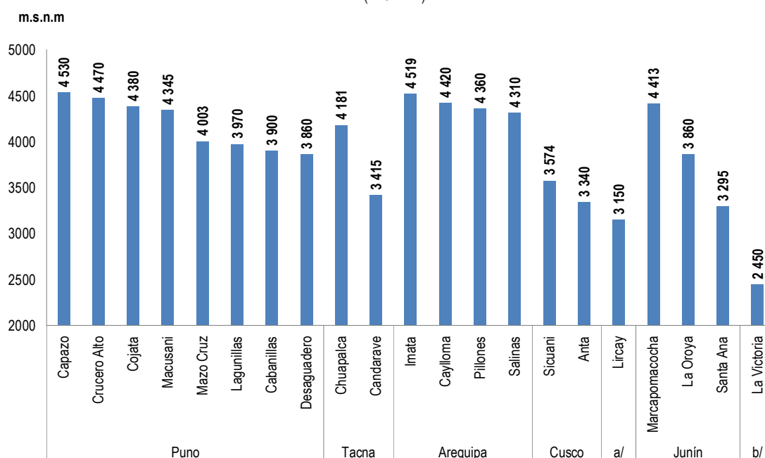
Gráfico N° 44 Perú: Altitud de las estaciones meteorológicas reportadas (m.s.n.m.)
