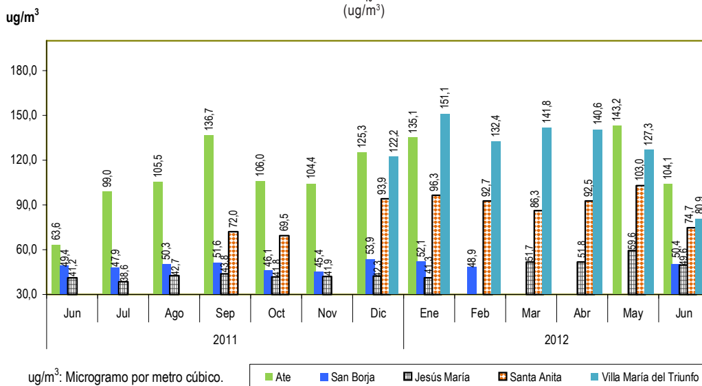
Gráfico N° 4 Lima Metropolitana: Valor mensual de PM 10 , por estaciones de medición, 2011-2012 (ug/m 3 )
