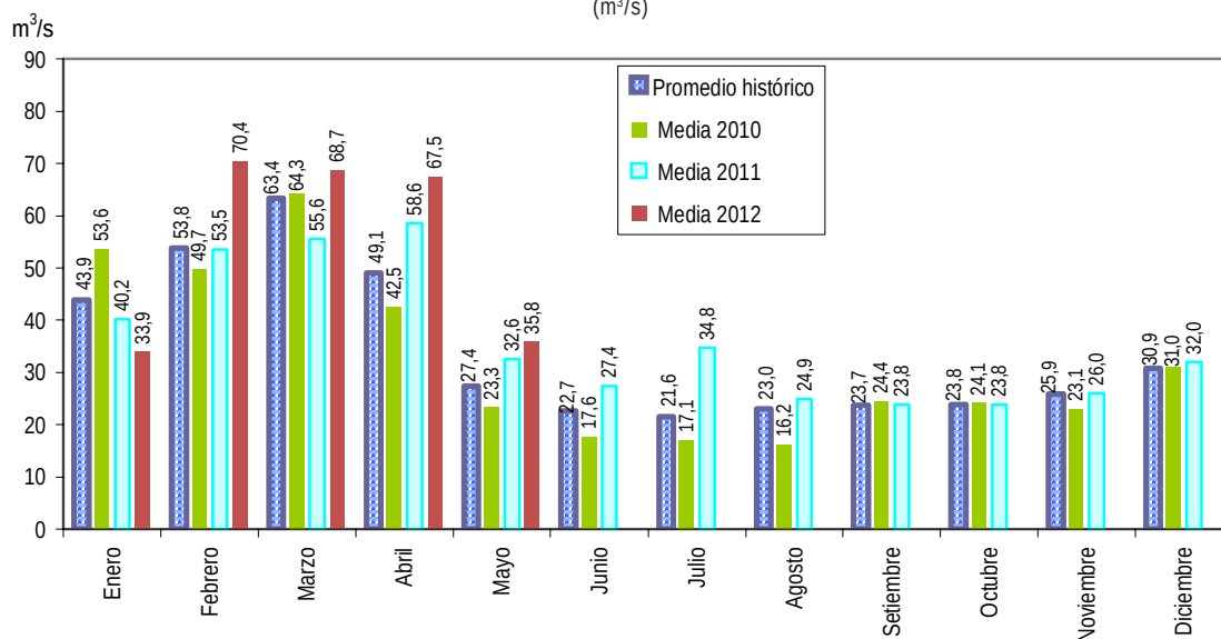
Gráfico N° 36 Lima Metropolitana: Caudal promedio y promedio histórico del río Rímac, 2010-2012 (m³/s)
