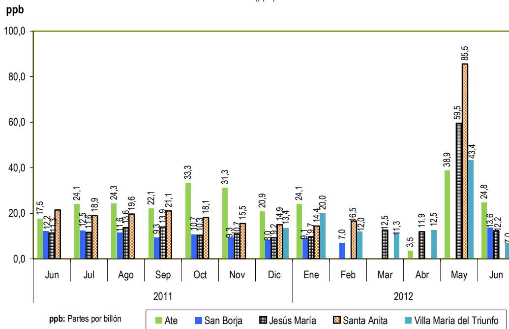
Gráfico N° 3 Lima Metropolitana: Valor mensual de Dióxido de Nitrógeno, por estaciones de medición, 2011-2012 (ppb)
