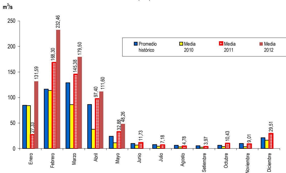
Gráfico N° 38 Perú: Caudal promedio de los ríos de la vertiente del Lago Titicaca, 2010-2012 (m 3 /s)
