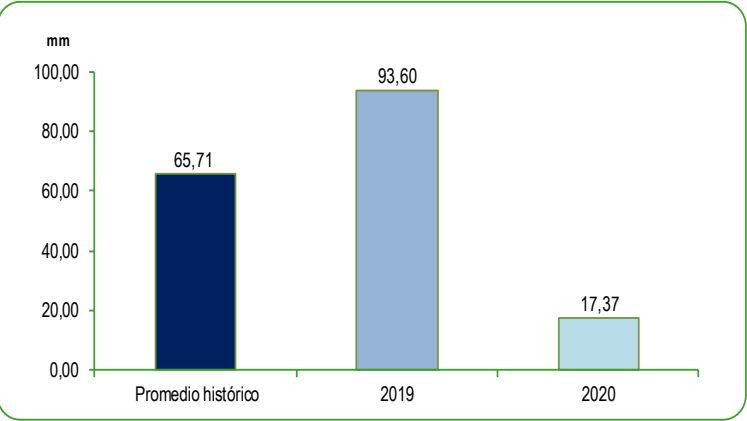
GRÁFICO N°41 PERÚ: PROMEDIO DE LAS PRECIPITACIONES EN LA VERTIENTE DEL LAGO TITICACA Mes: Noviembre 2019 - 2020 Milímetros (mm)
