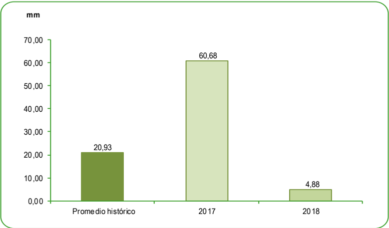
GRÁFICO N° 57 PERÚ: PROMEDIO DE LAS PRECIPITACIONES EN LA VERTIENTE DEL LAGO TITICACA Mes: Setiembre 2017 - 2018 Milímetros (mm)
