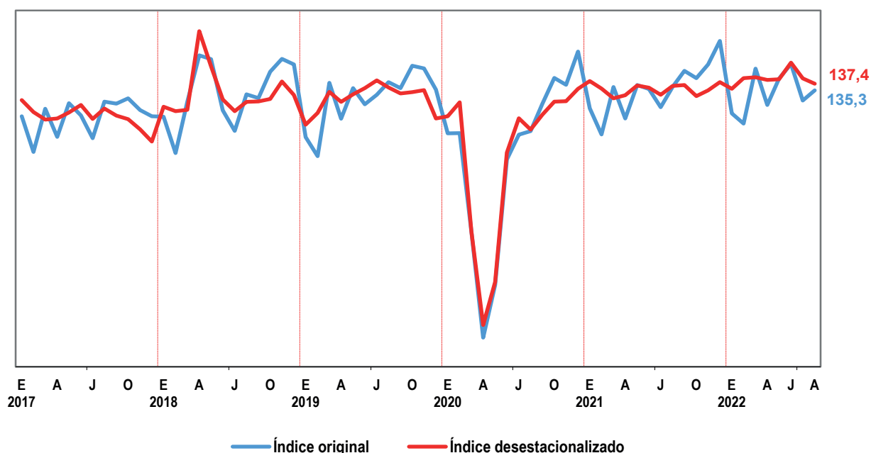
Gráfico N° 07 Evolución Mensual del Índice Original y Desestacionalizado del Sector Manufactura: 2017-2022 (Año base: 2007=100,0)
