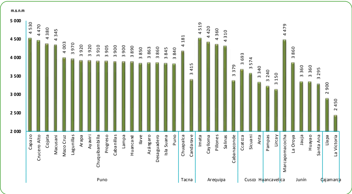
GRÁFICO N°35 PERÚ: ALTITUD DE LAS ESTACIONES METEOROLÓGICAS Metros sobre el nivel del mar
