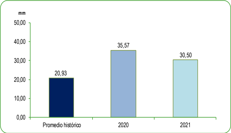
GRÁFICO N°31 PERÚ: PROMEDIO DE LAS PRECIPITACIONES EN LA VERTIENTE DEL LAGO TITICACA Mes: Setiembre 2020 - 2021 Milímetros (mm)
