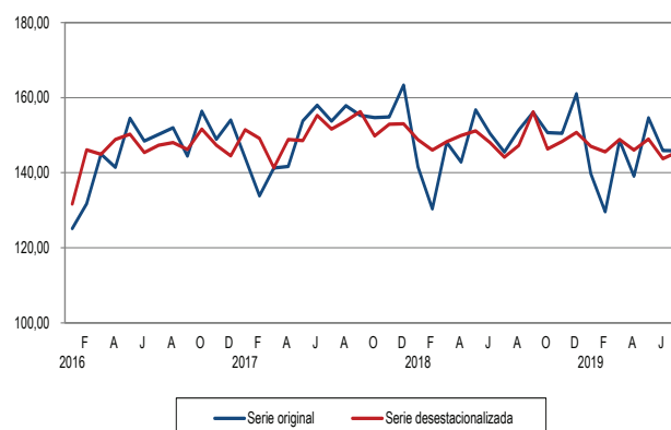
Índice de la Producción Minera y de Hidrocarburos Año base 2007 Serie original y desestacionalizada Enero 2016-Julio 2019
