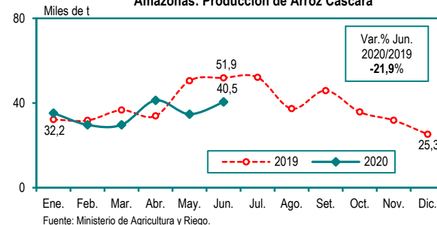
Amazonas: Producción de Arroz Cáscara
