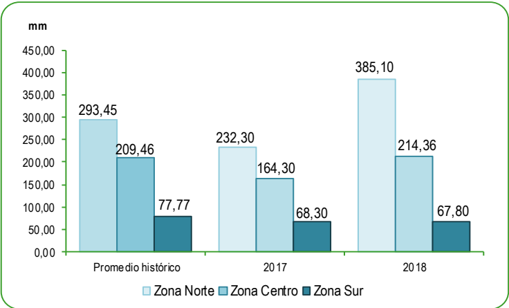
GRÁFICO N° 74 PERÚ: PROMEDIO DE LAS PRECIPITACIONES EN LA VERTIENTE DEL ATLÁNTICO Mes: Diciembre 2017 - 2018 Milímetros (mm)
