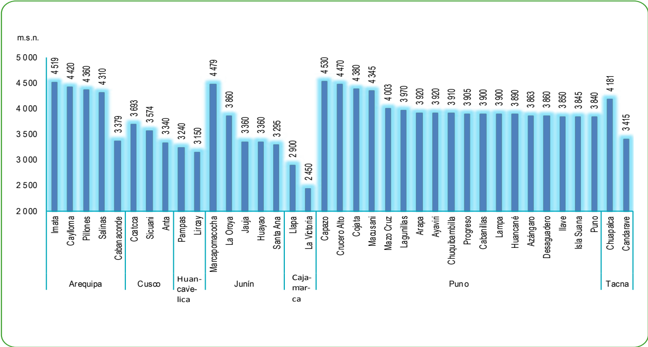
GRÁFICO N° 79 PERÚ: ALTITUD DE LAS ESTACIONES METEOROLÓGICAS Metros sobre el nivel del mar
