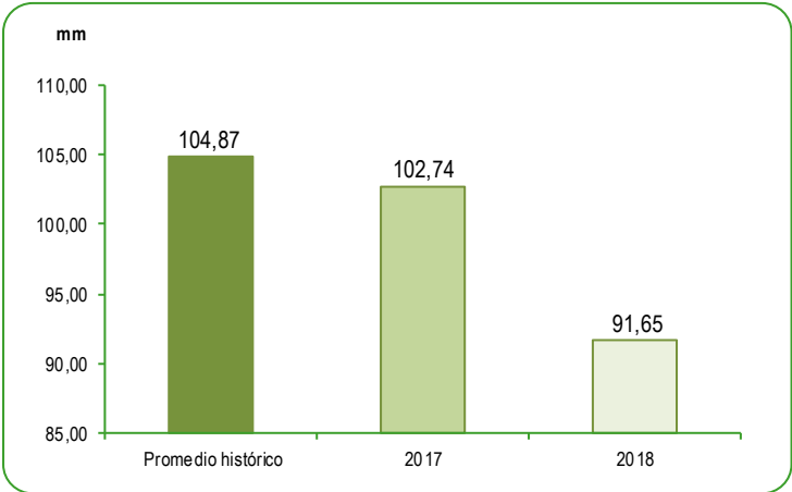
GRÁFICO N° 75 PERÚ: PROMEDIO DE LAS PRECIPITACIONES EN LA VERTIENTE DEL LAGO TITICACA Mes: Diciembre 2017 - 2018 Milímetros (mm)
